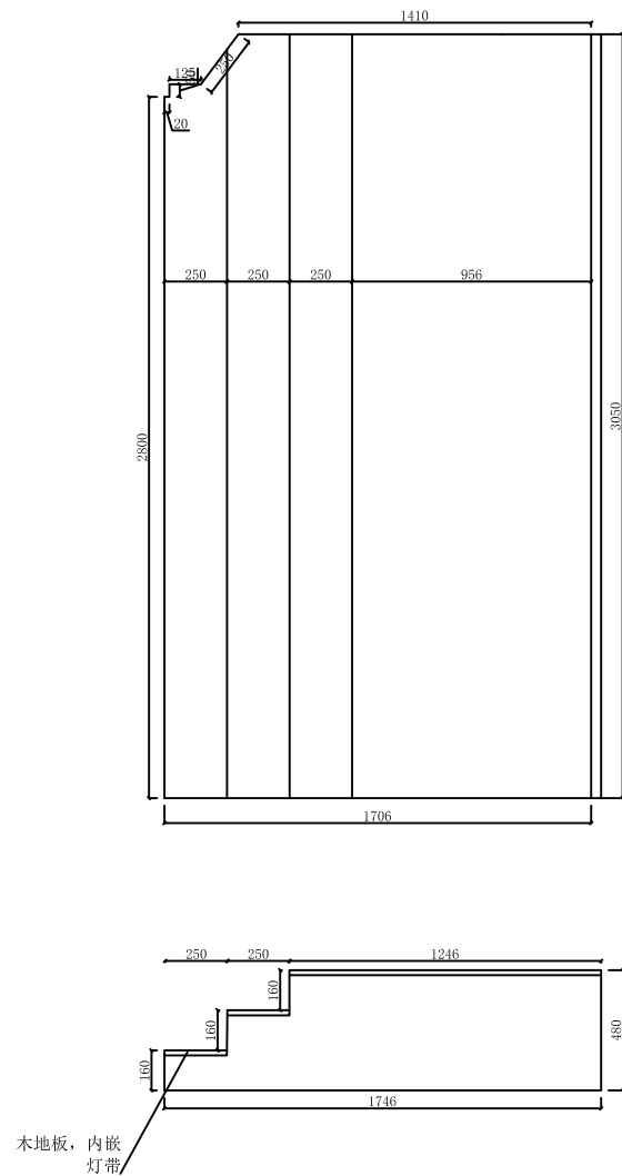
台阶立面图
