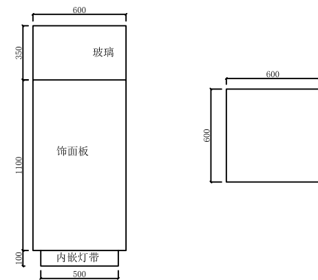
展台尺寸图
