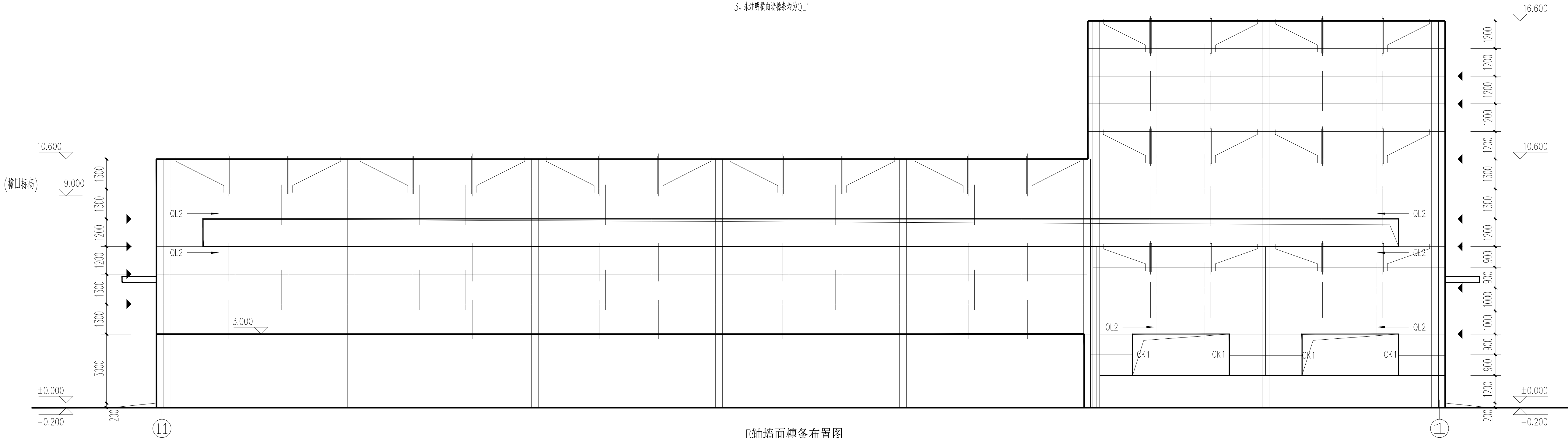
E轴墙面標条布置图
