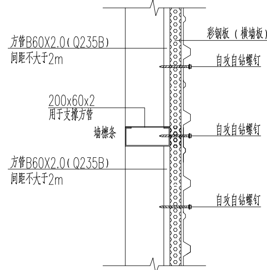
墙面板安装示意图
