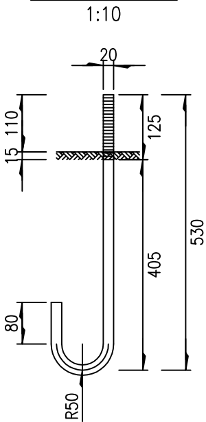
地脚螺栓大样图
