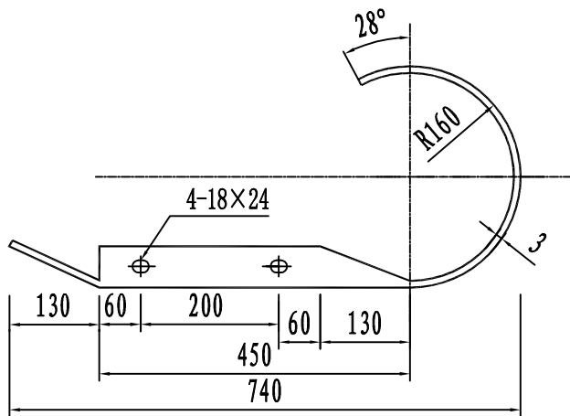
普通护栏端头 D-I 平面图 1:10
