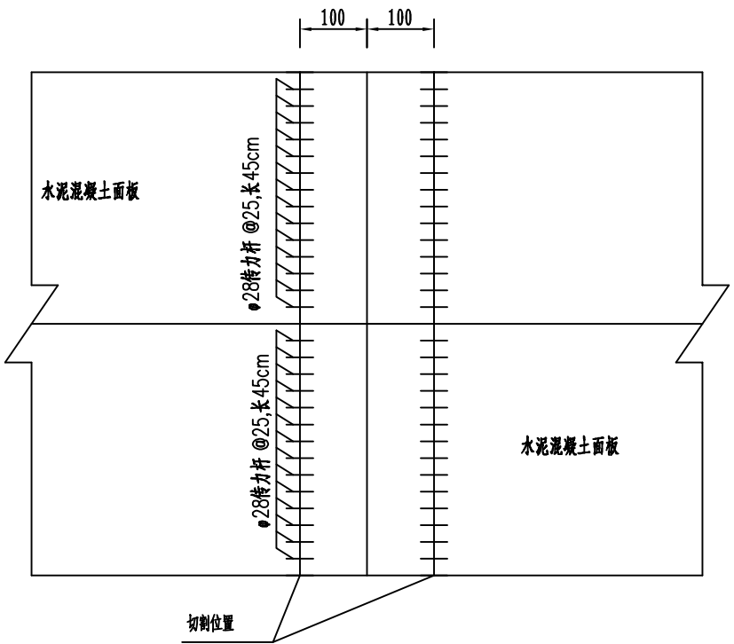
胀缝维修大样图
