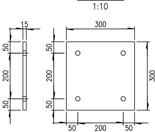
基础法兰盘
