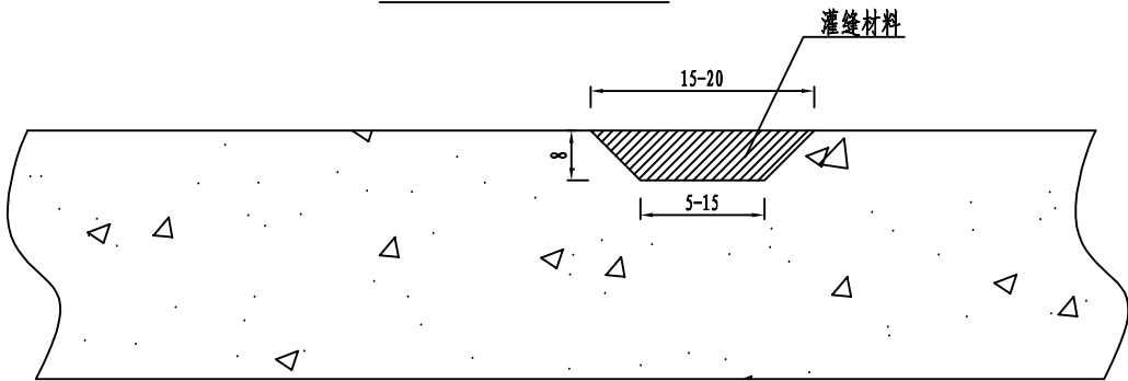
条带灌浆(单位:mm)
