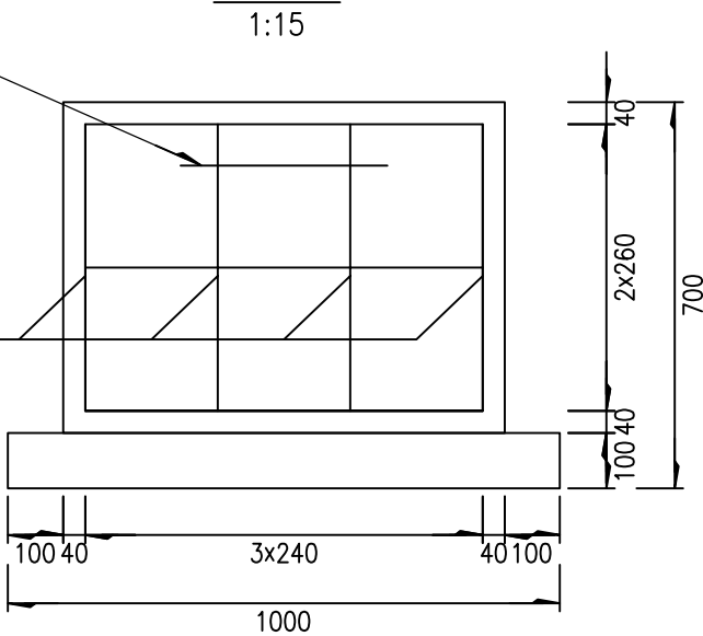
侧面图
