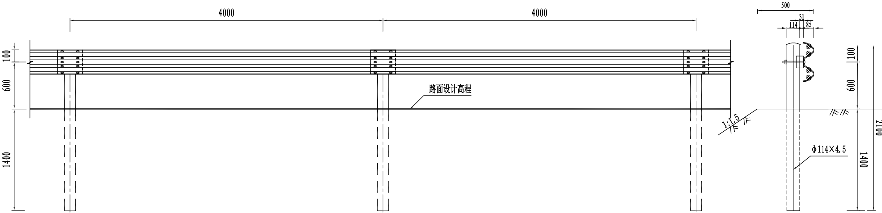
Gr-C-4E护栏立面图 1: 30
