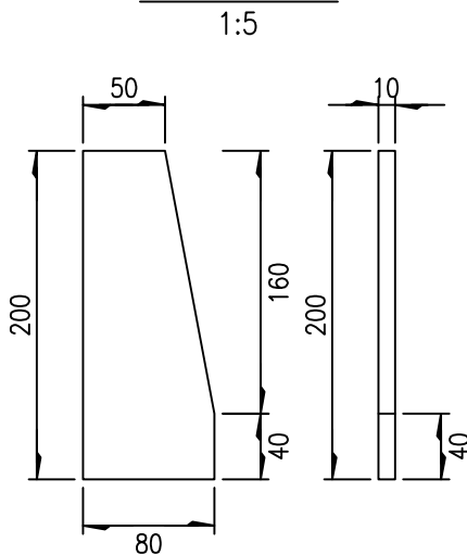
加劲肋构造图
