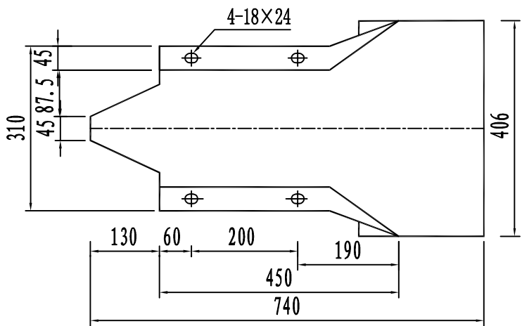
普通护栏端头 D-I 立面图 1:10
