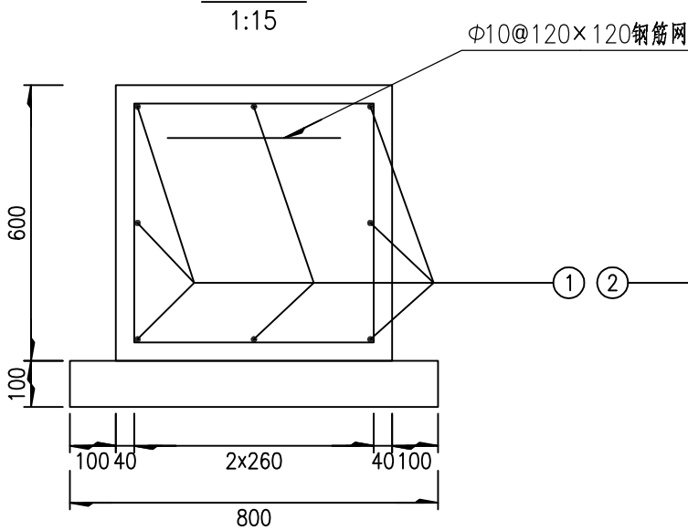
立面图
