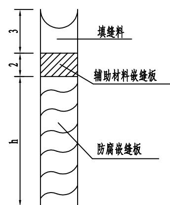
胀缝放大图
