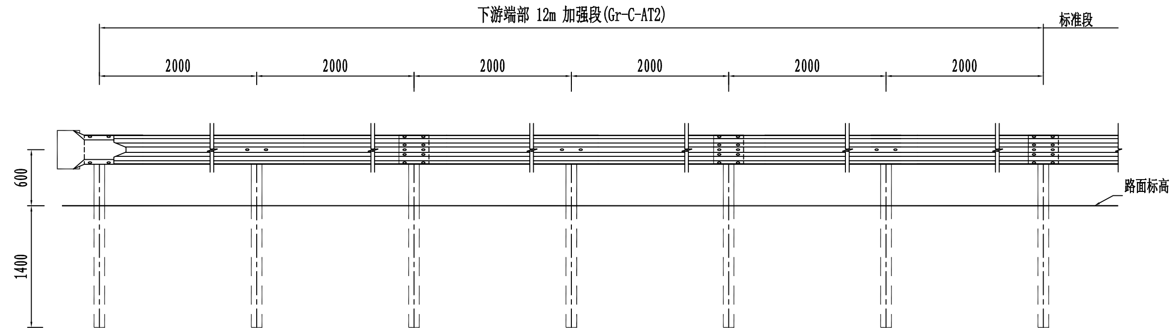
下游端头立面图 1:40
