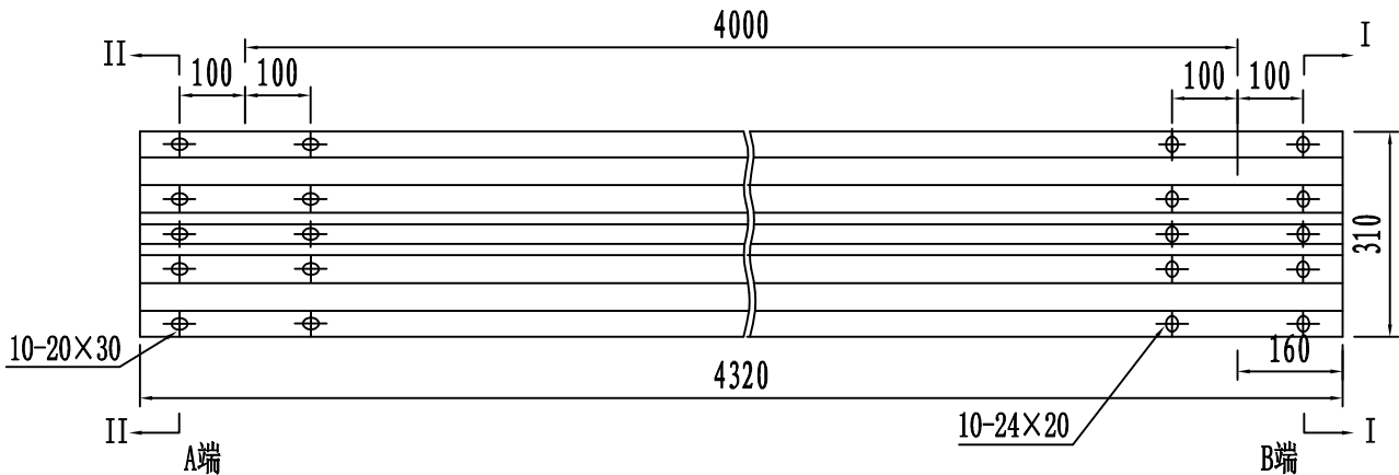
立面图 1:6 DB01-1
