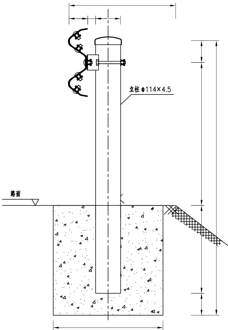
侧面图 1:10 Gr-C-4C
