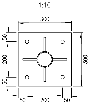
加劲法兰盘
