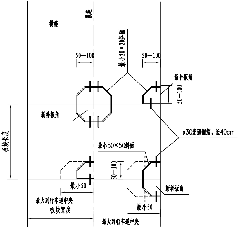
修补板角大样图
