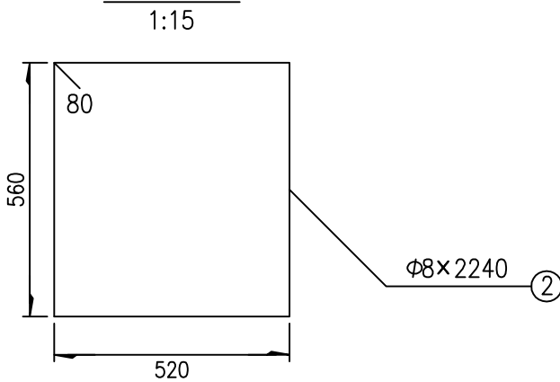
箍筋大样图
