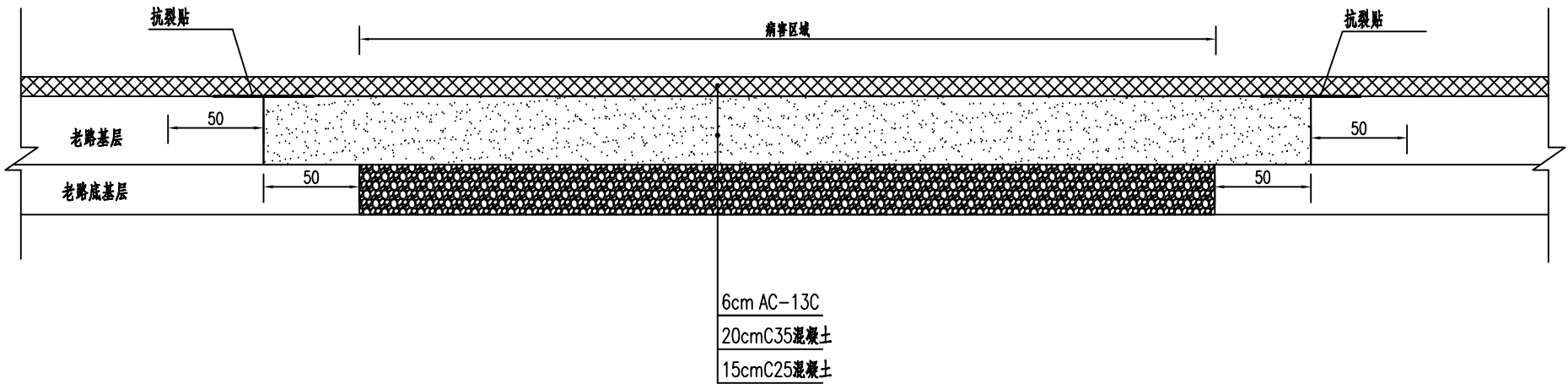
局部坑槽、沉陷处理断面示意图
