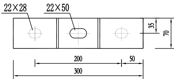
托架 1:5 (300×70×4.5)
