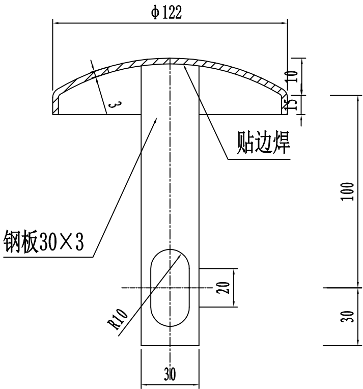
柱帽大样图 1:2
