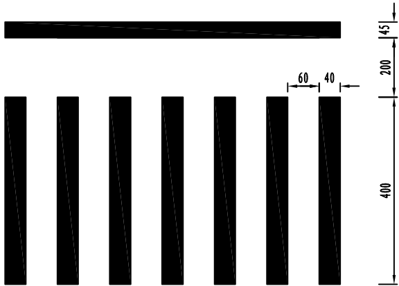
人行横道线大样图 1: 100
