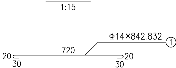
主筋大样图
