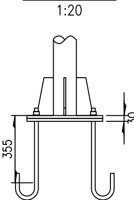
基础连接大样
