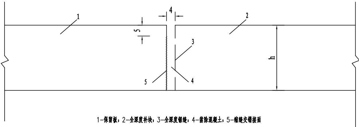
集料嵌锁法(单位:cm)
