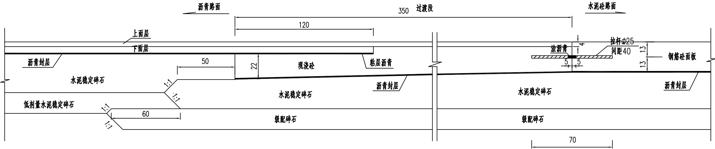
刚性路面与柔性路面连接图
