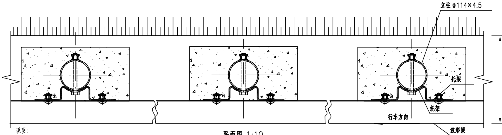
平面图 1:10 Gr-C-4C
