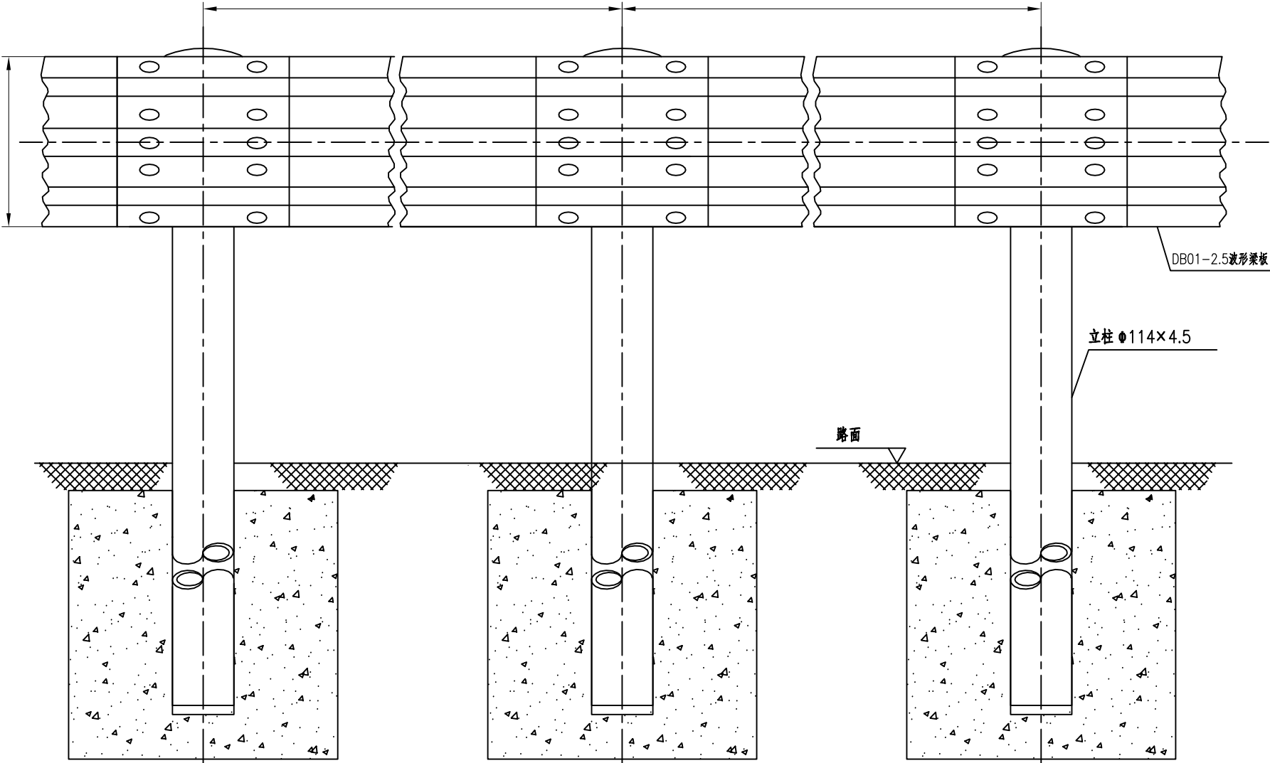
立面图 1:10 Gr-C-4C
