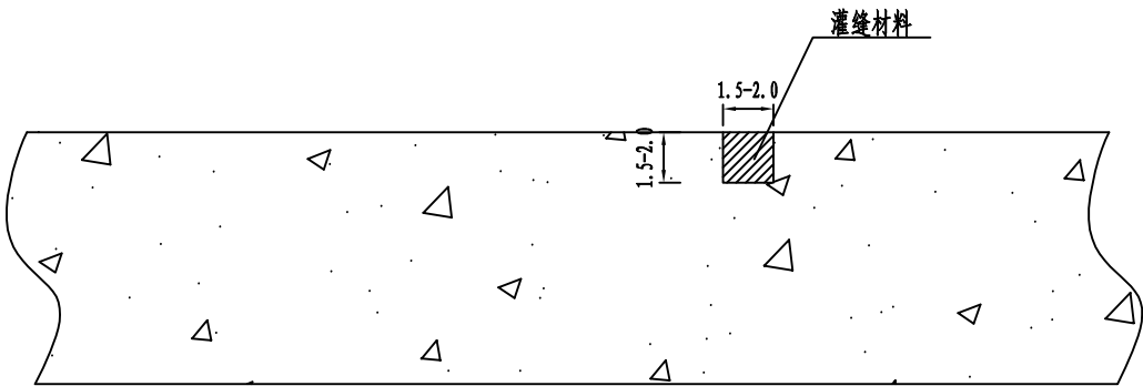
扩缝灌浆(单位:mm)
