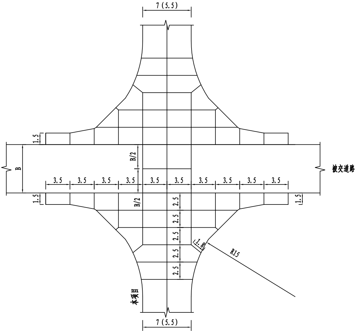
典型十字交叉口水泥板块划分示意图
