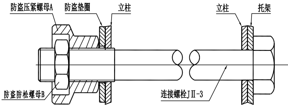
C节点大样图 1:1
