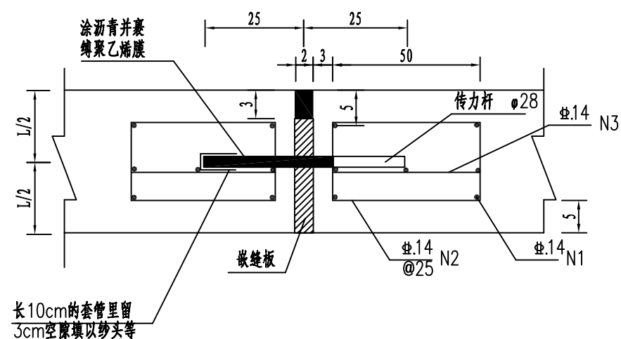
胀缝构造图
