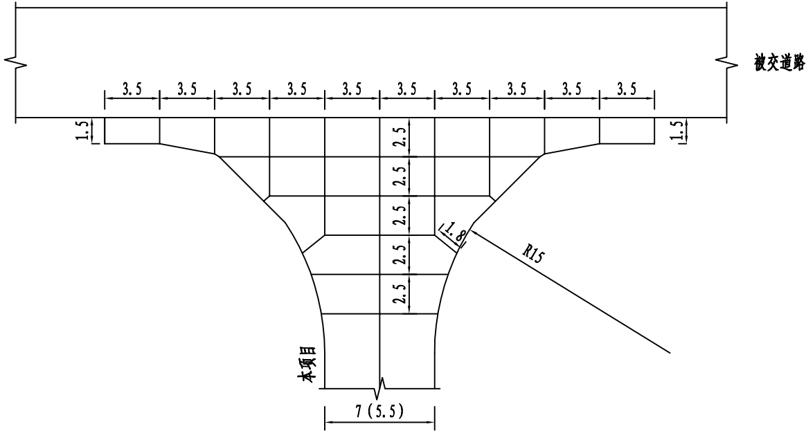
典型T字交叉口水泥板块划分示意图
