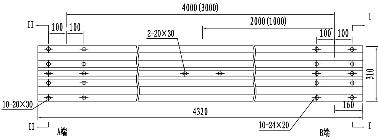
立面图 1:6 DB01-2( DB03)
