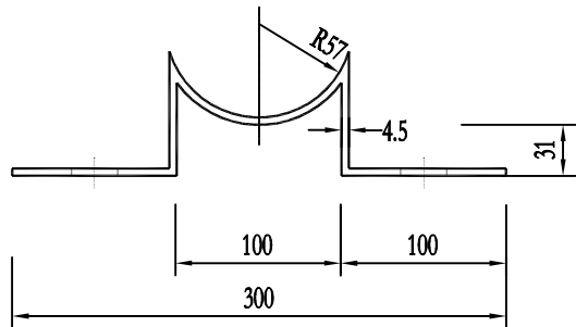
托架 1:5 (300×70×4.5)
