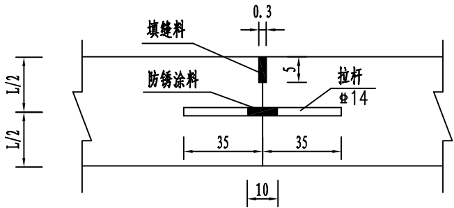
纵向施工缝横断面
