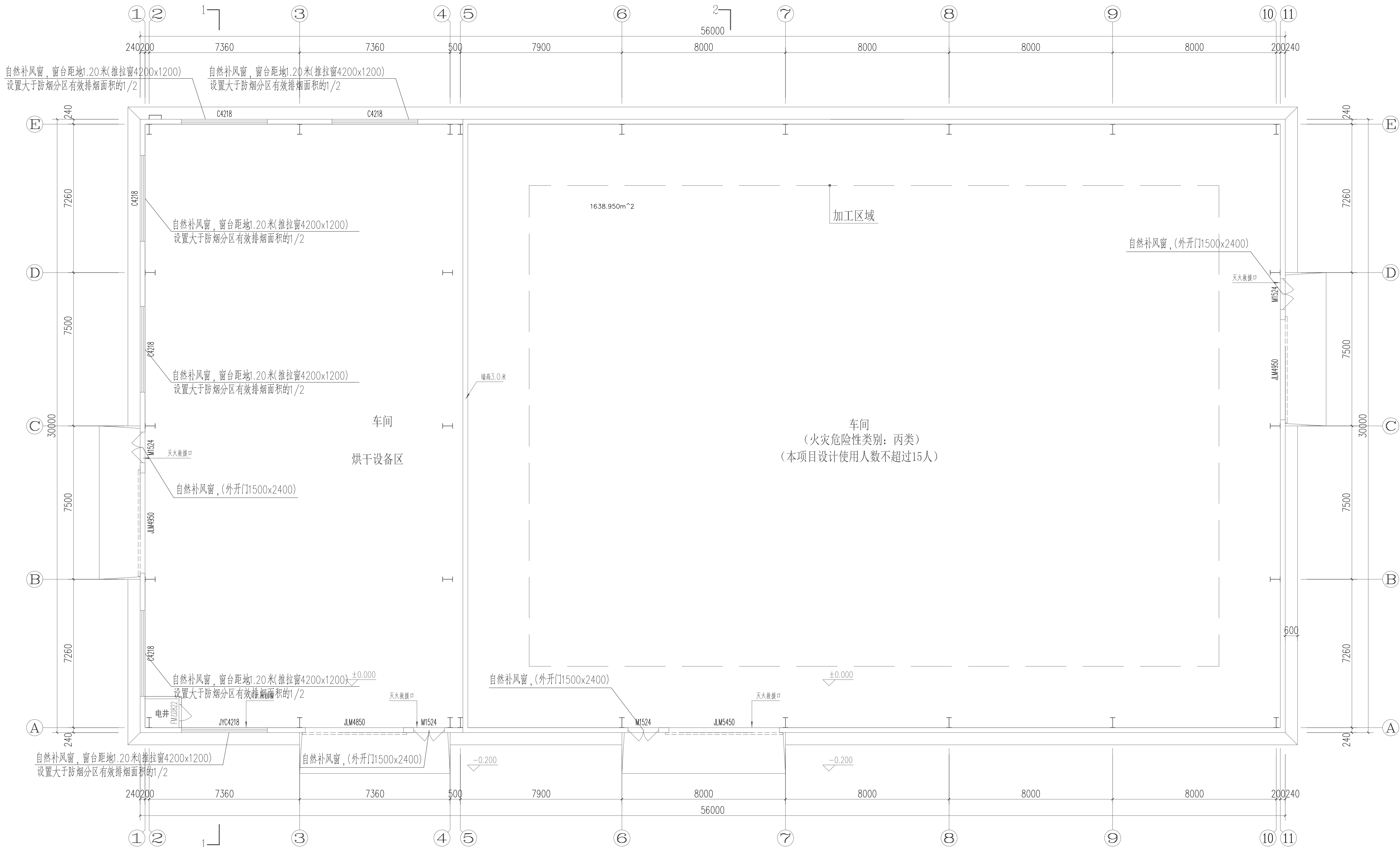
一层通风平面图 1:100
