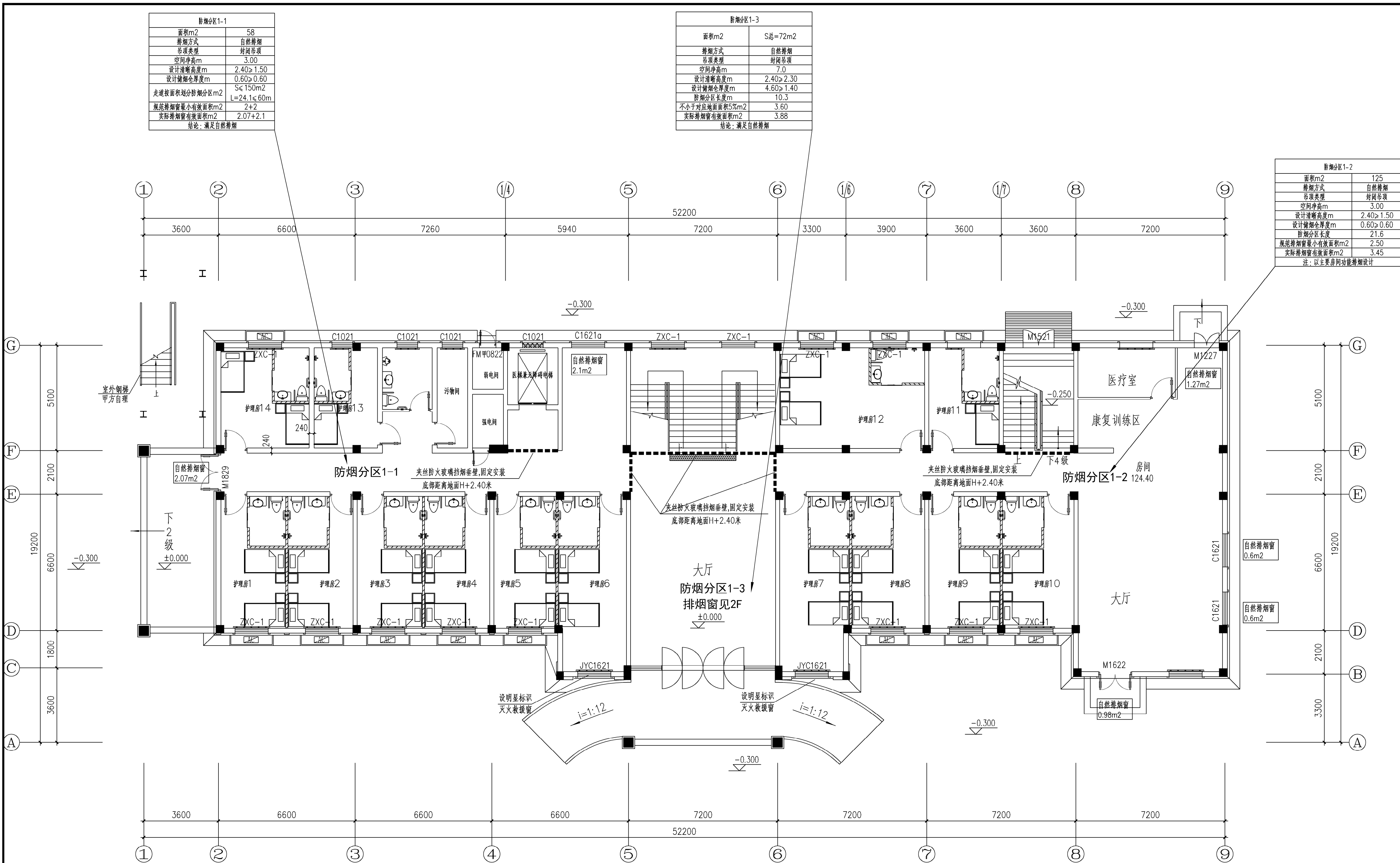
一层消防报审防排烟平面图 1:100
