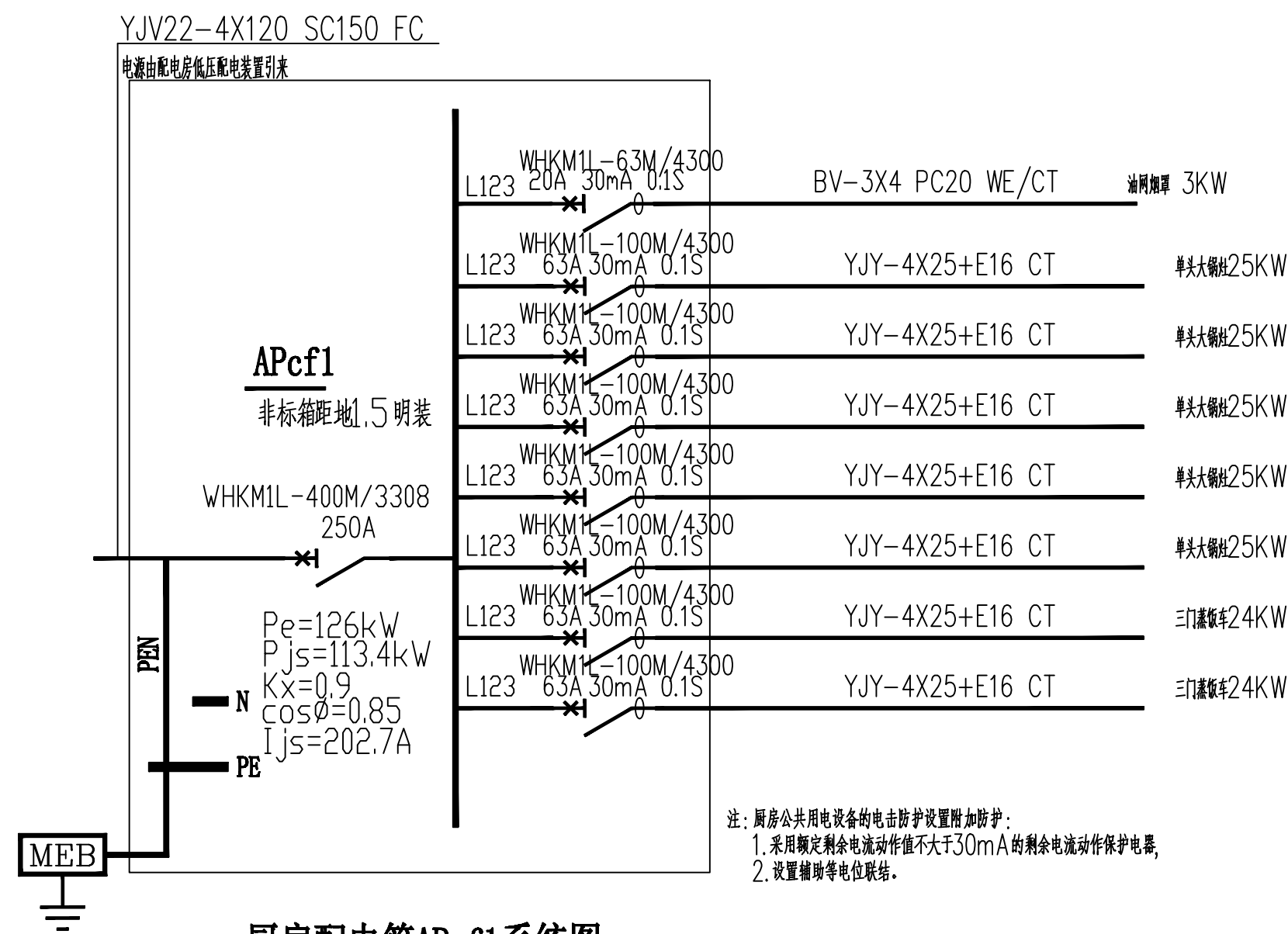
厨房配电箱APcf1系统图
