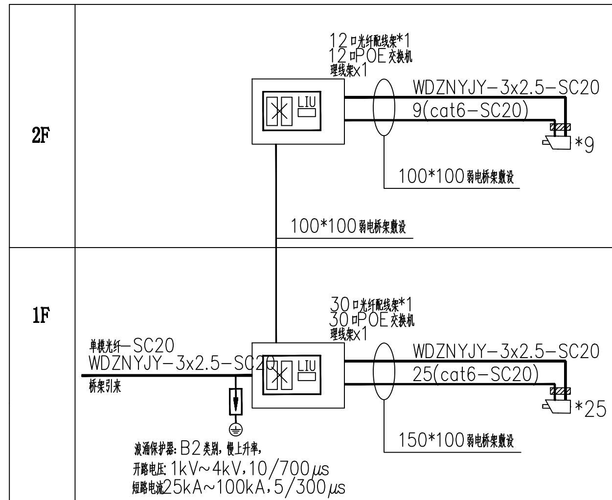
食堂监控系统图
