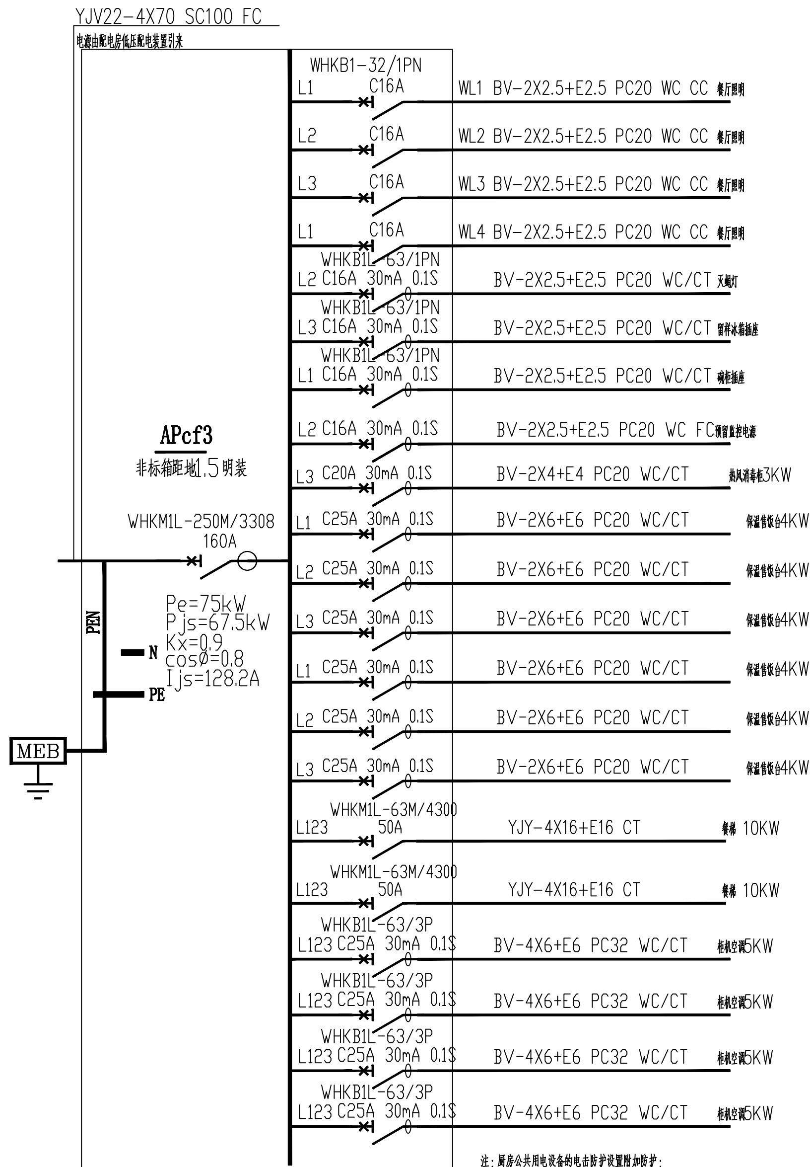
厨房配电箱APcf3系统图
