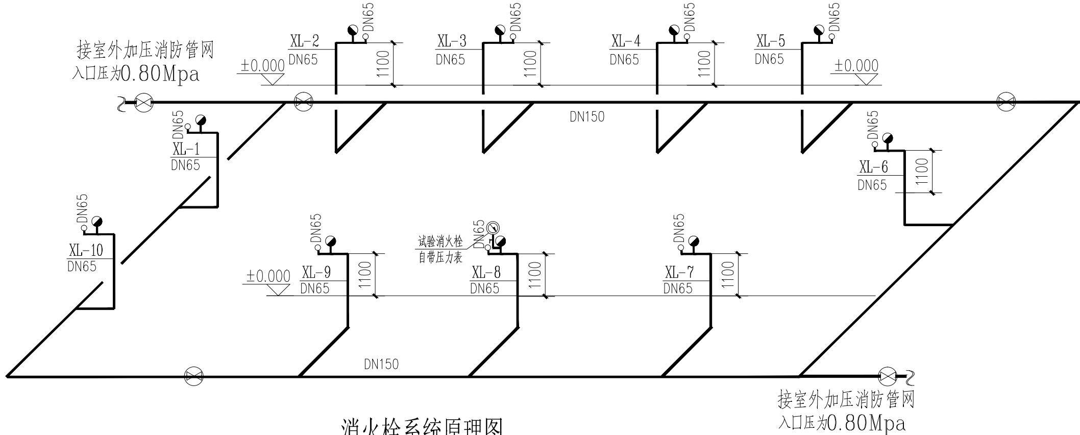
消火栓系统原理图
