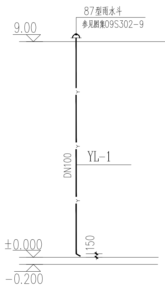
雨水系统原理图
