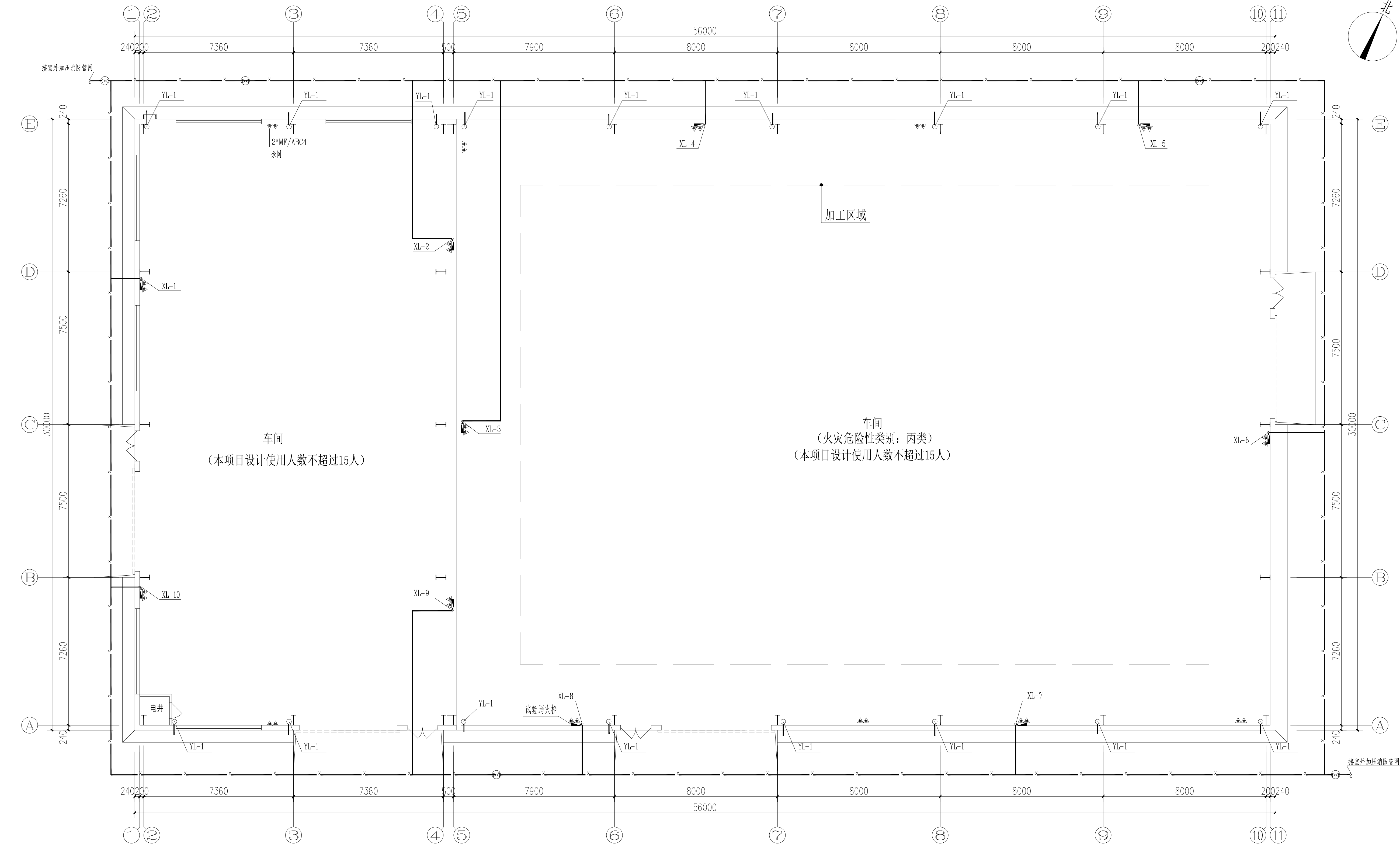
一层给排水平面图 1:100
