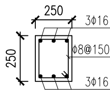
过梁配筋图
