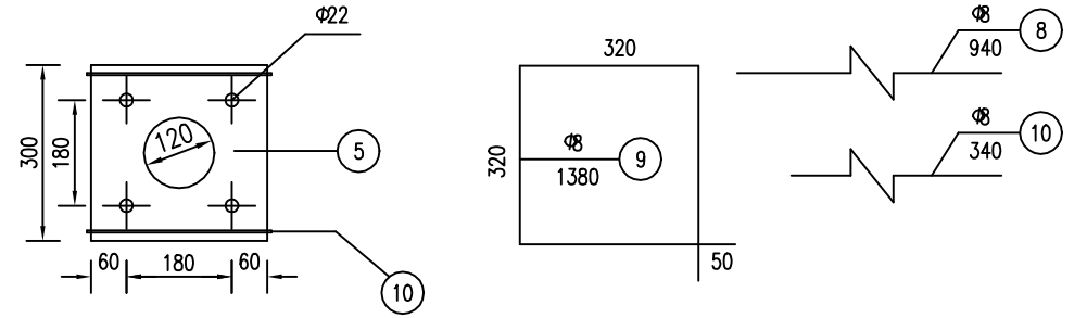
材料数量表
