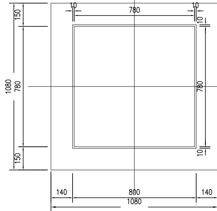
窨井座平面图 1:15
