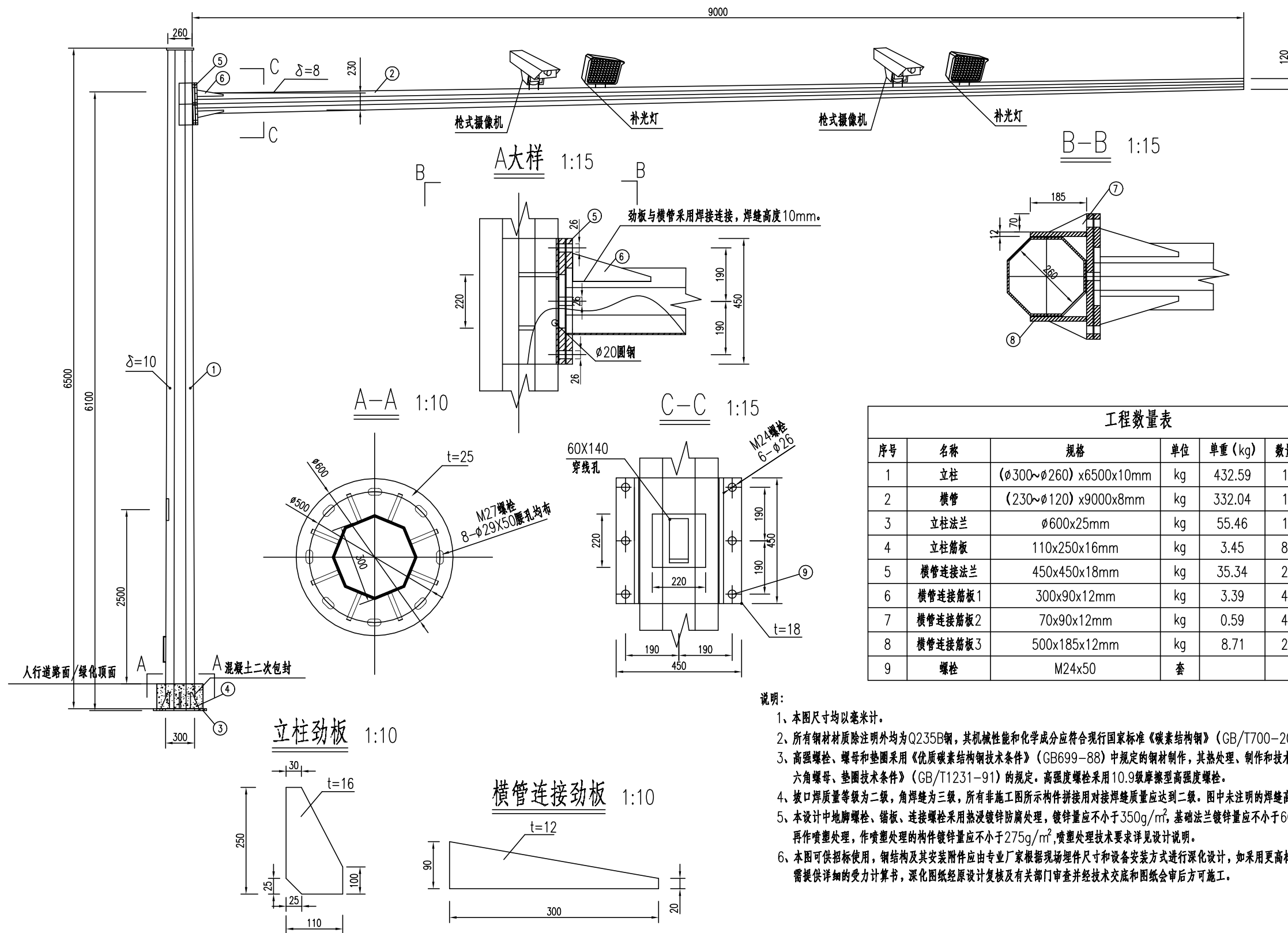
立面图 1:50
