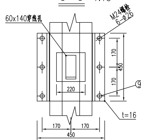
C-C 1:15
