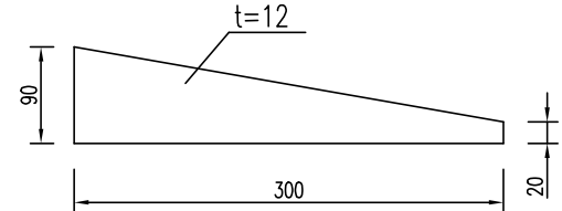
横管连接劲板 1:10
