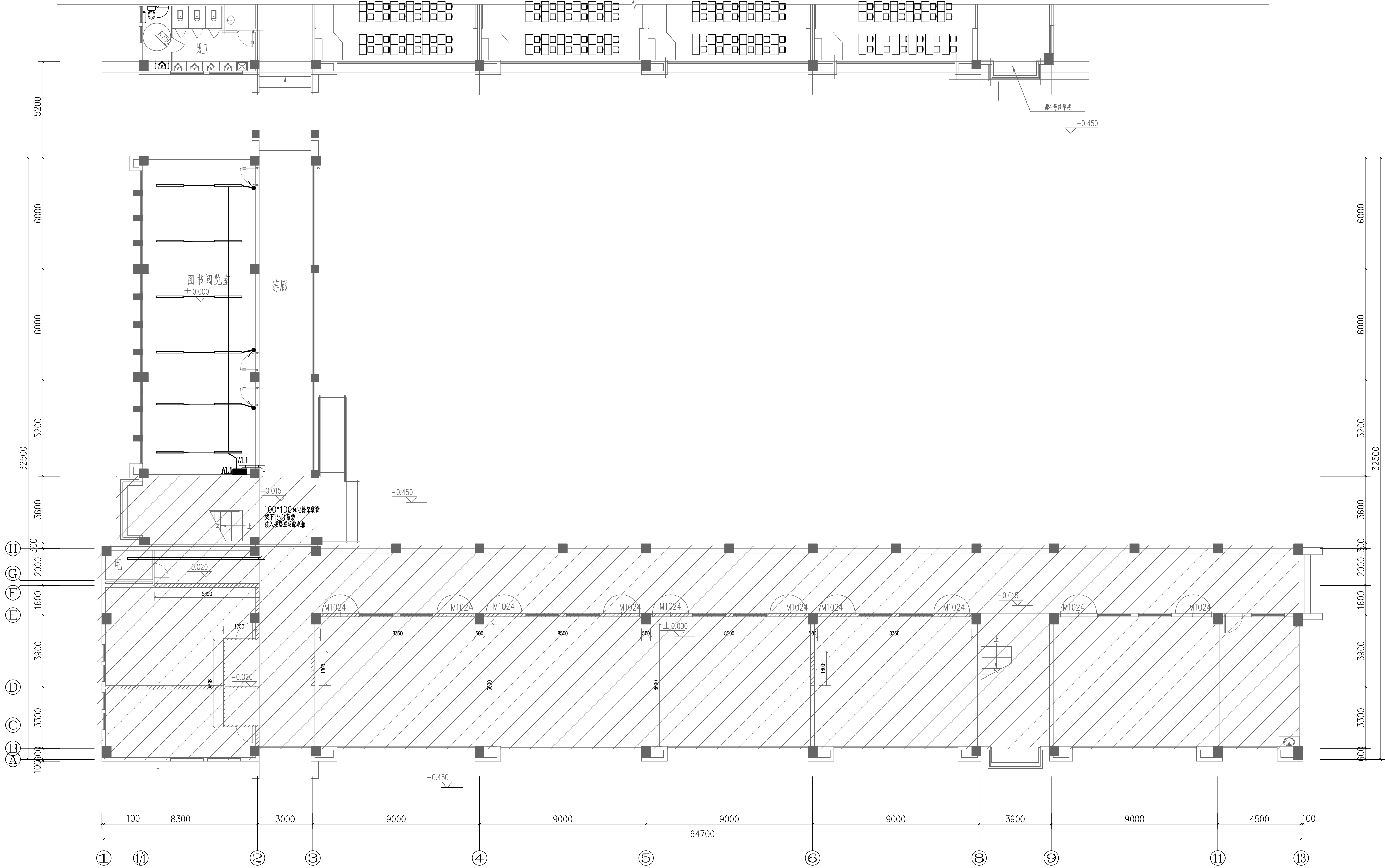
一层照明平面图 1:100
