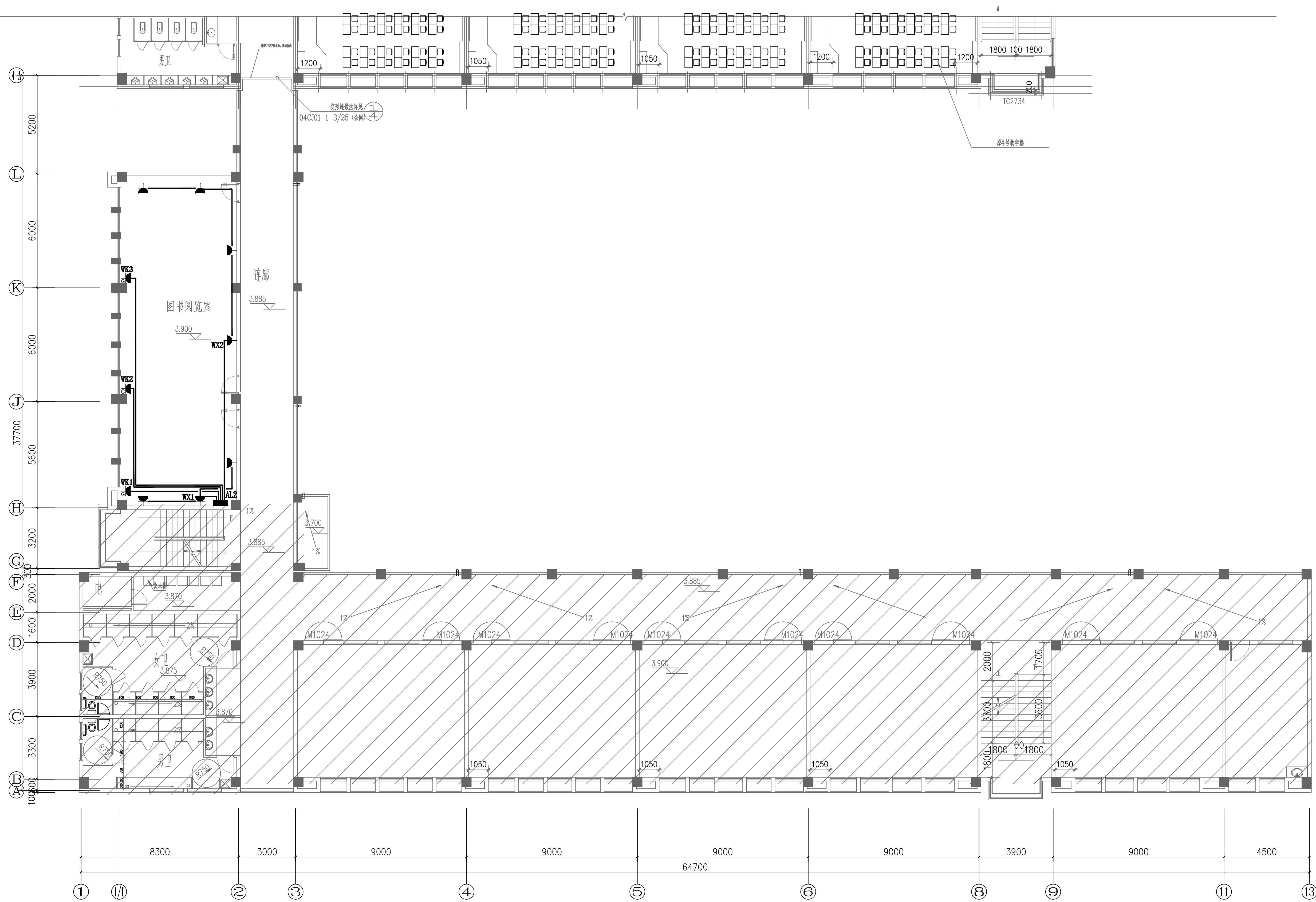
二层插座平面图 1:100
