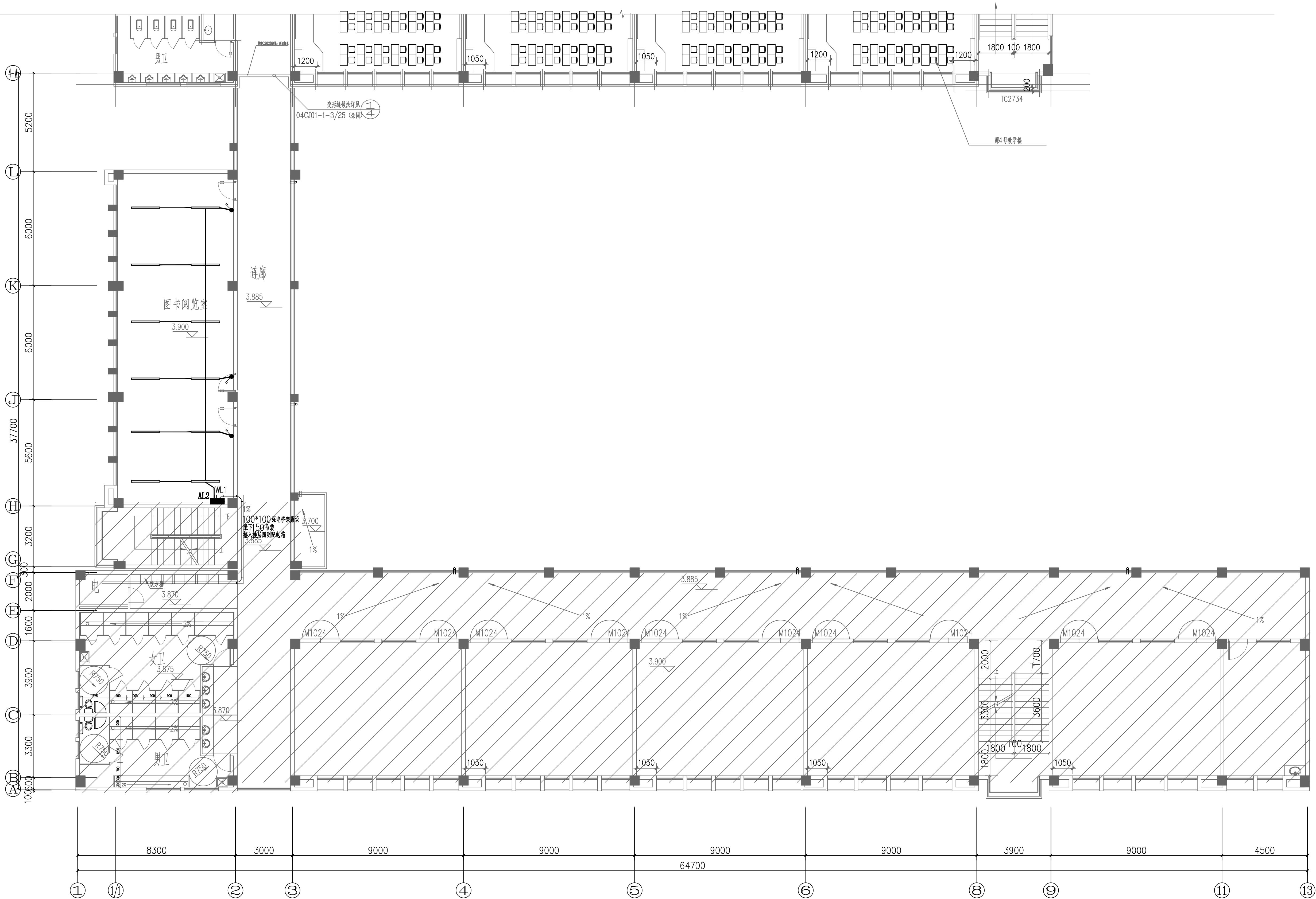
二层照明平面图 1:100
