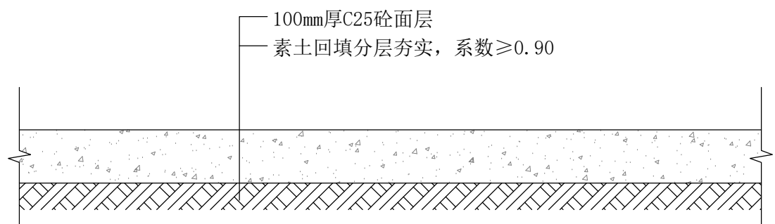
4 垃圾分类亭地面做法剖面图 1:10 注: 场地位置由甲方确定, 地面长约3米, 宽约1.2米
