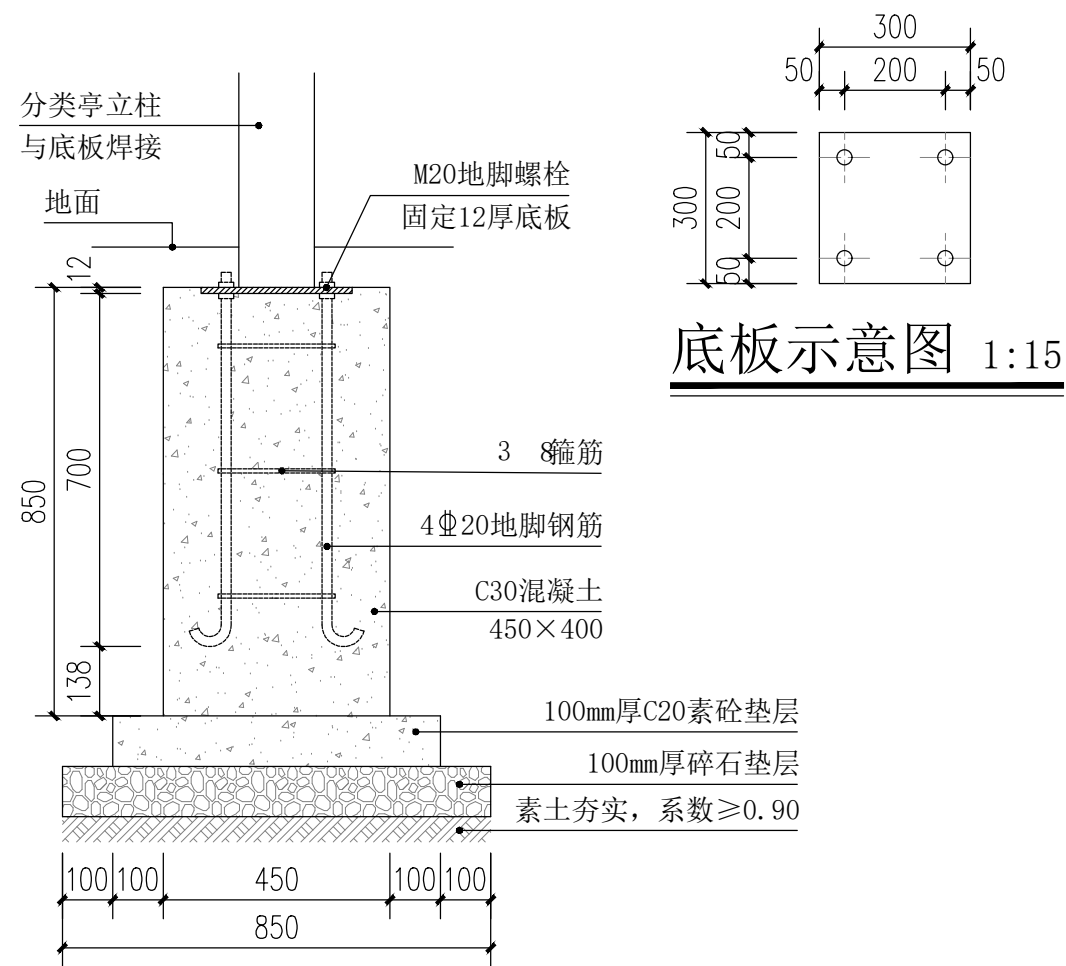
5 垃圾分类亭基础做法 1:15
