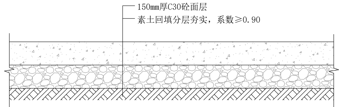
1 移动卫生间场地铺装做法剖面图 1:10 铺装尺寸为: 5.7m×2.7m
