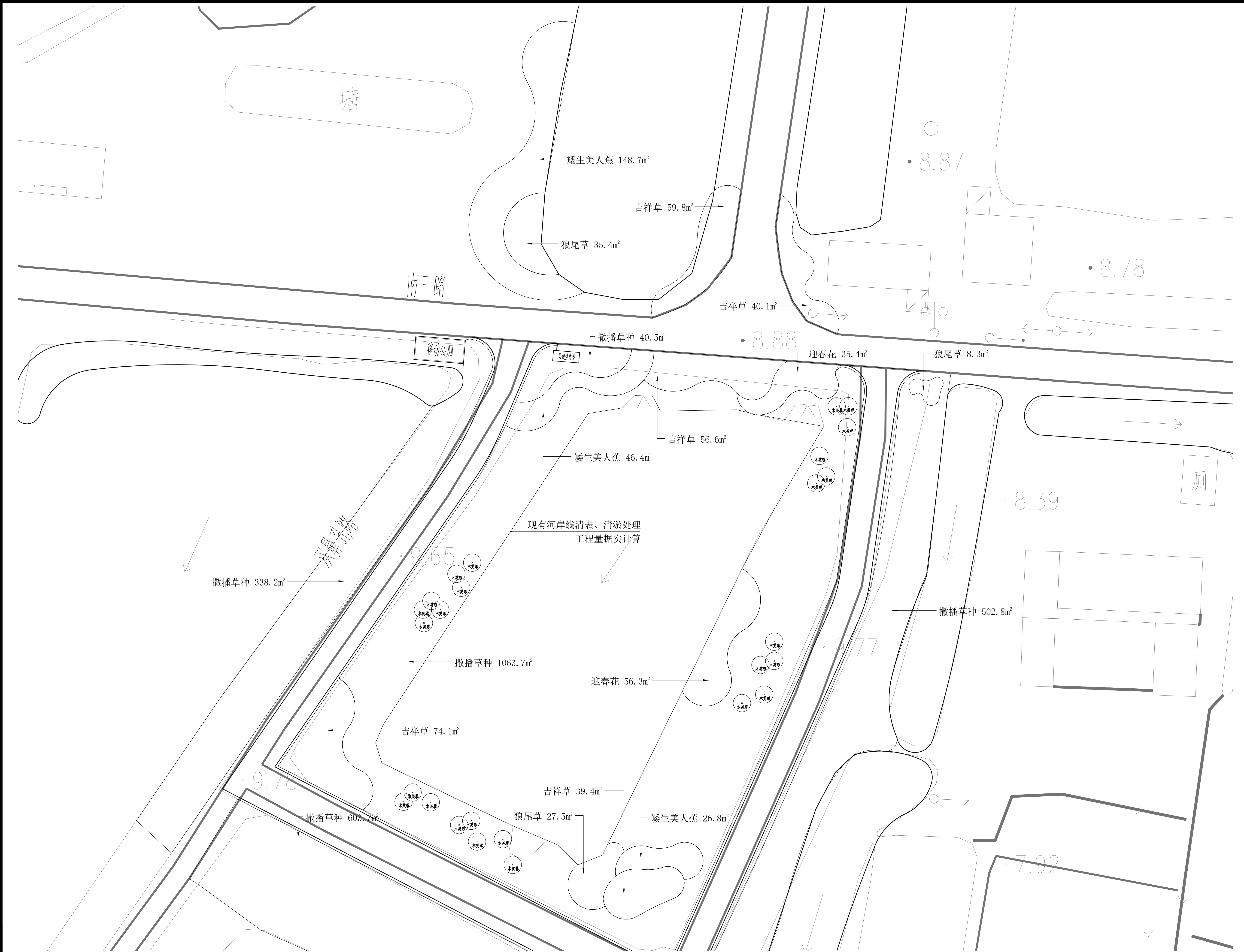
双鼻孔路景观节点平面图 1:200
