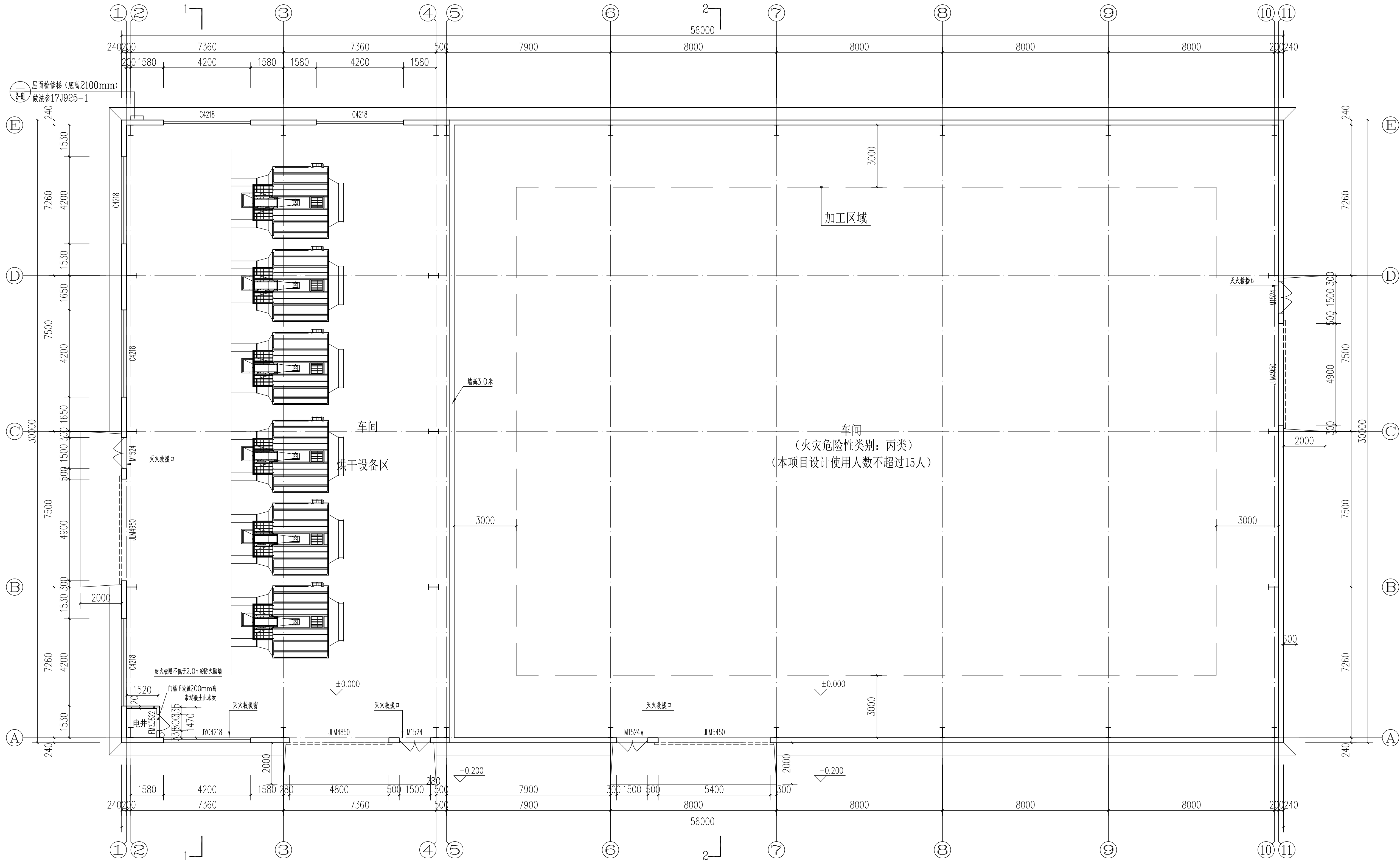
一层平面图 1:100
