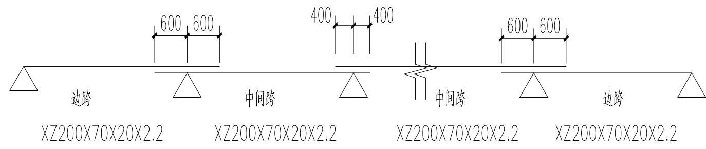
连续檩条搭接长度示意图 Q355B连续檩条
