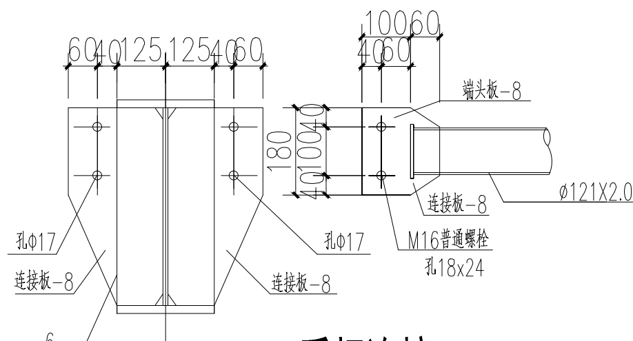
系杆连接
