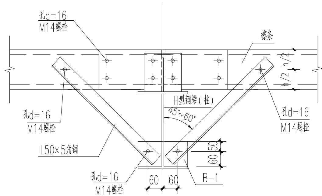
双面角隅撑
