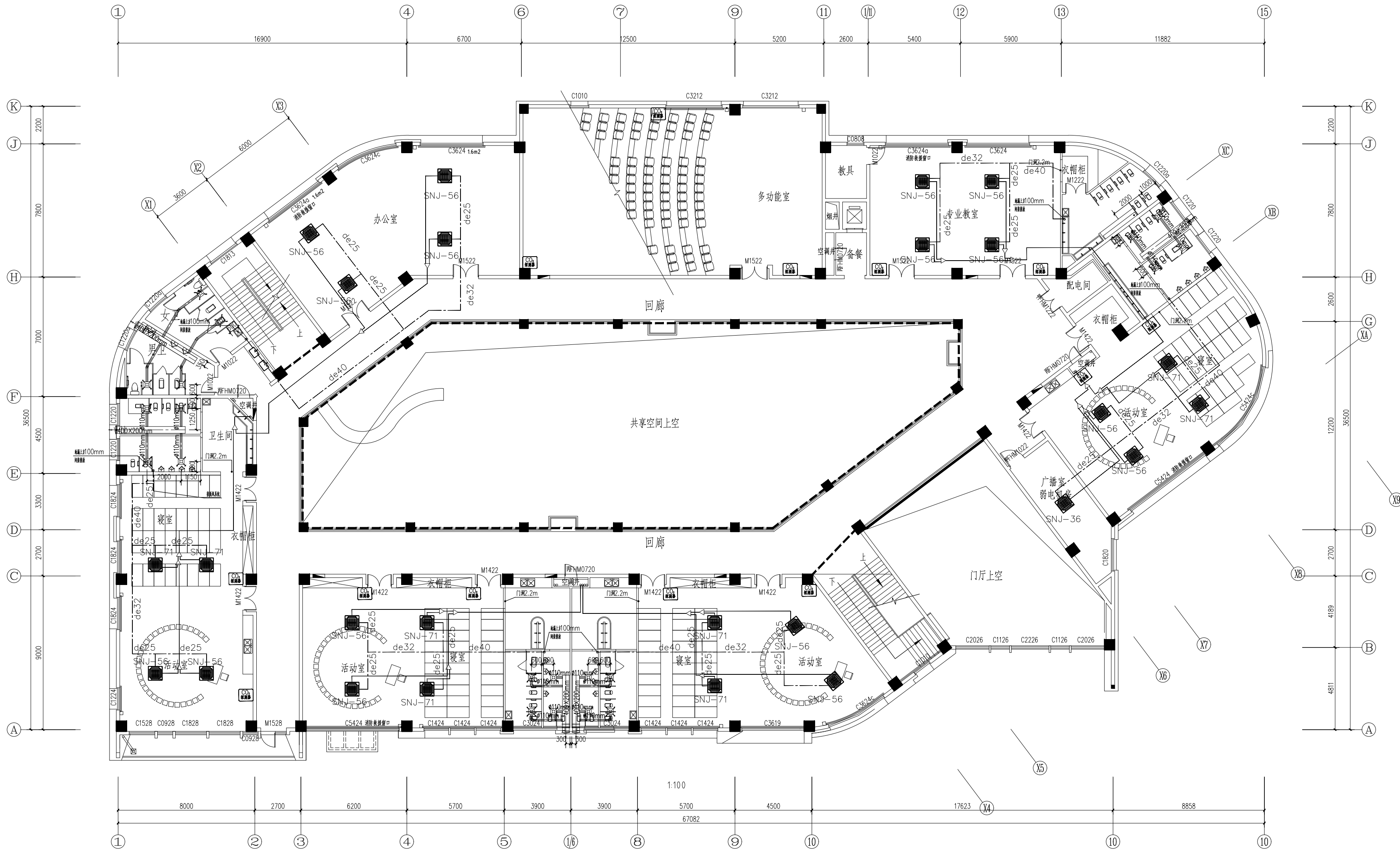
二层空调平面图
