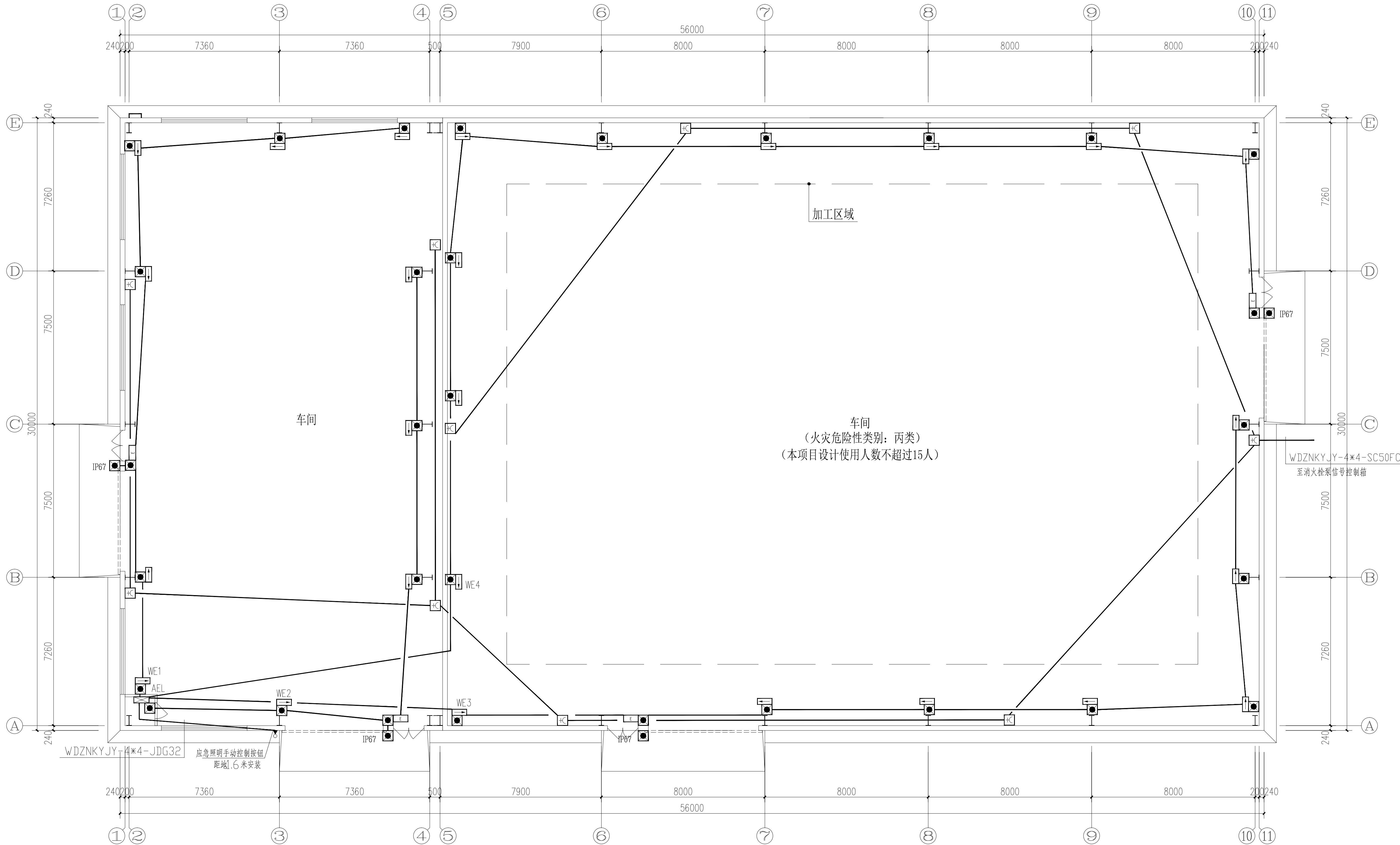
一层应急照明及疏散指示平面图 1:100
