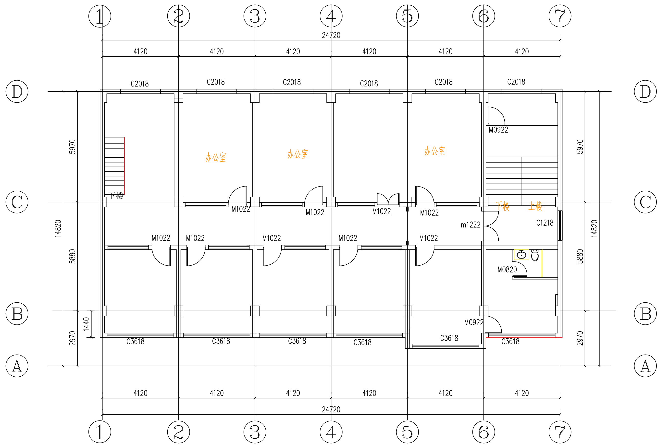
二层平面布置图 1:100
