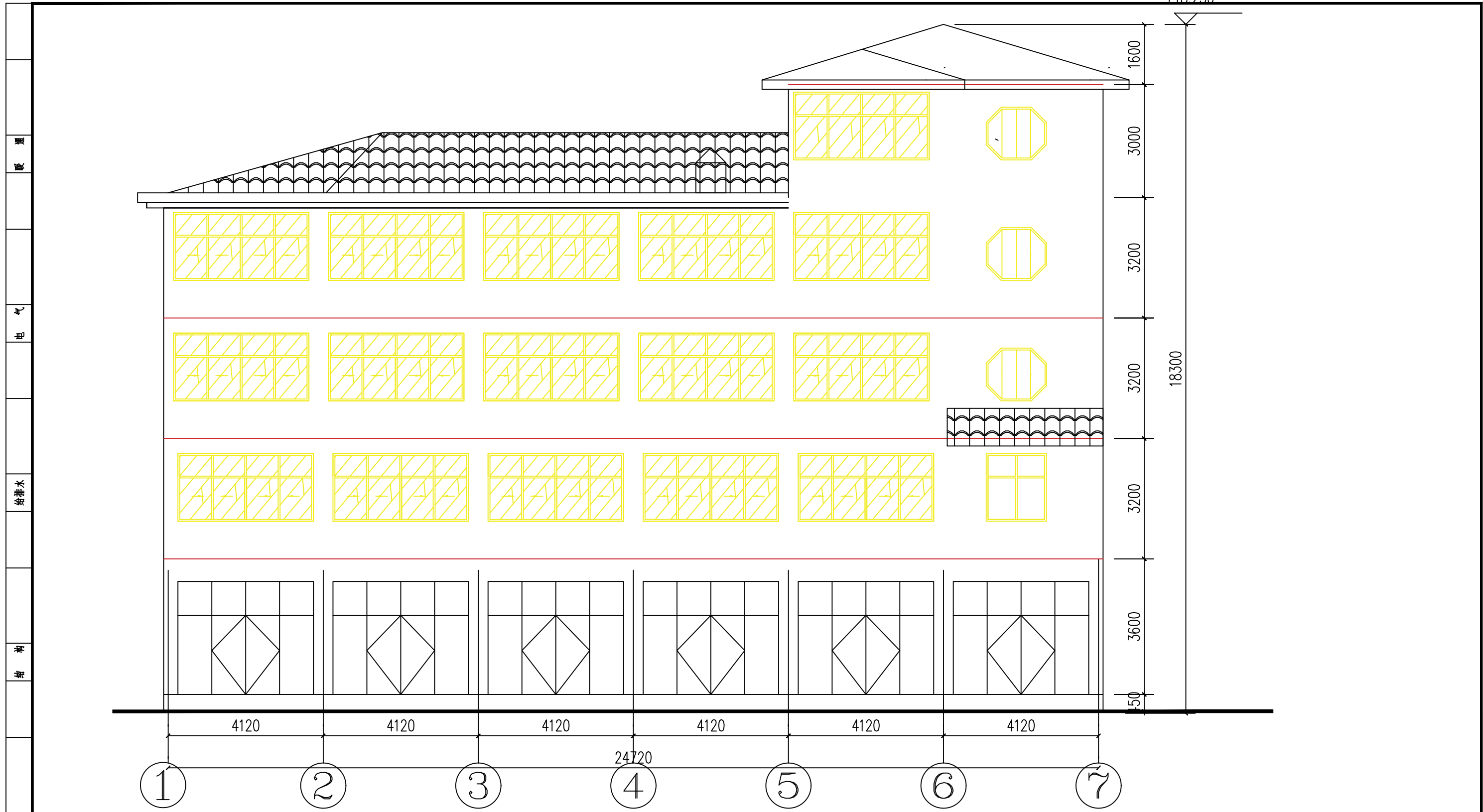
①—⑦ 轴立面图 1:150
