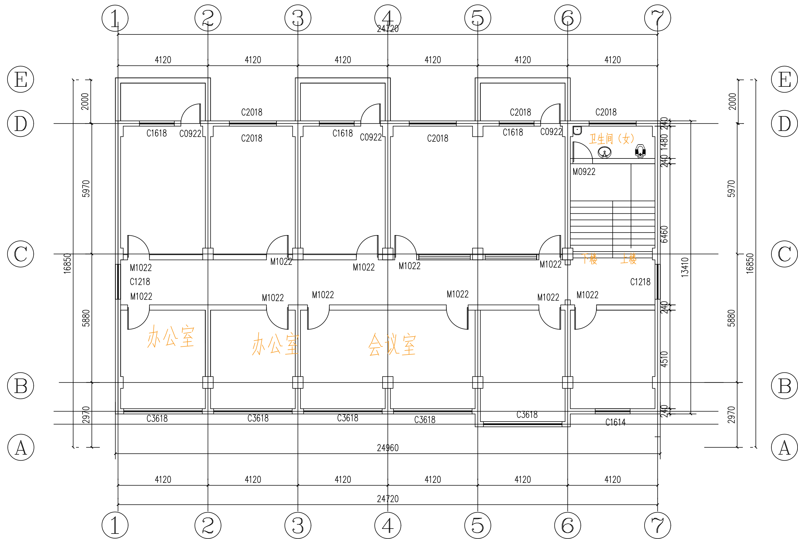
三层平面布置图 1:100
