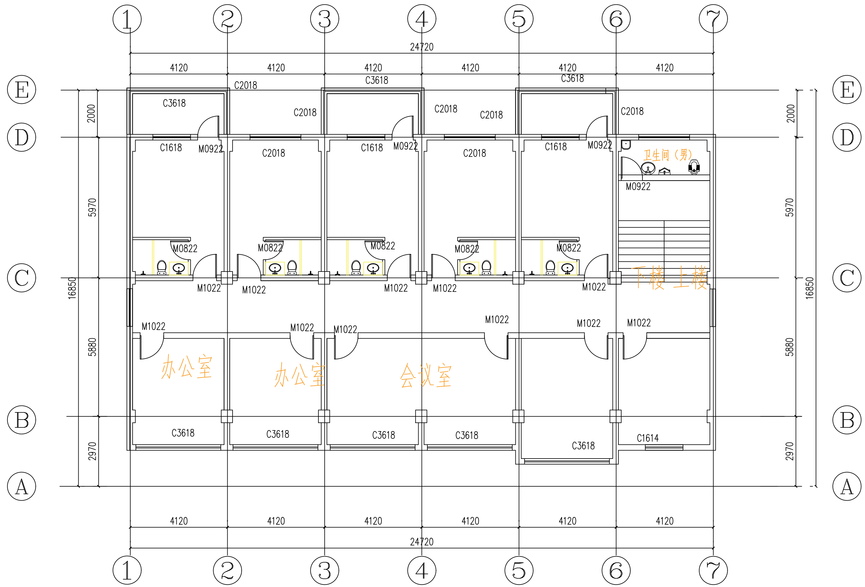
四层平面布置图 1:100
