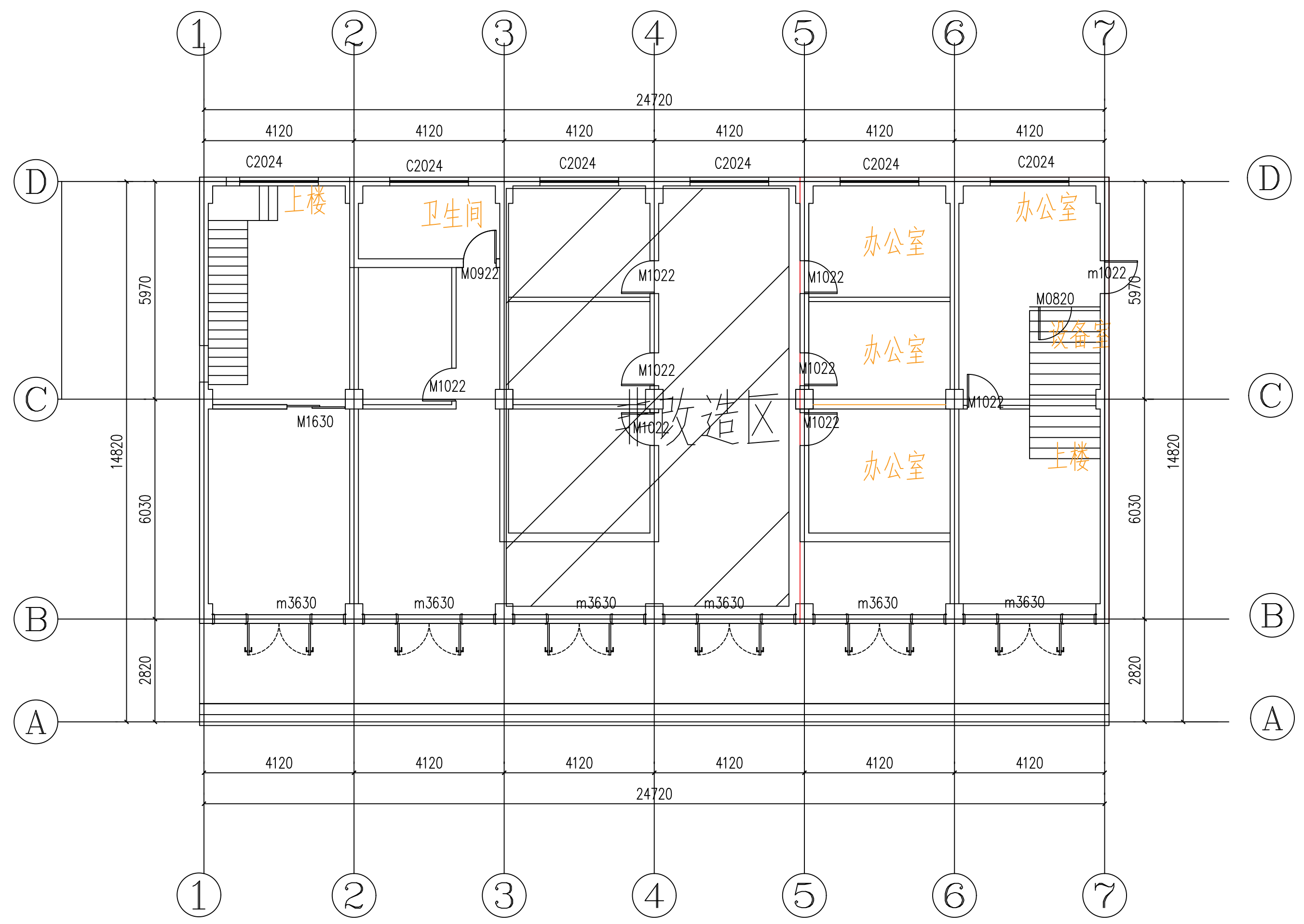
一层平面布置图 1:150
