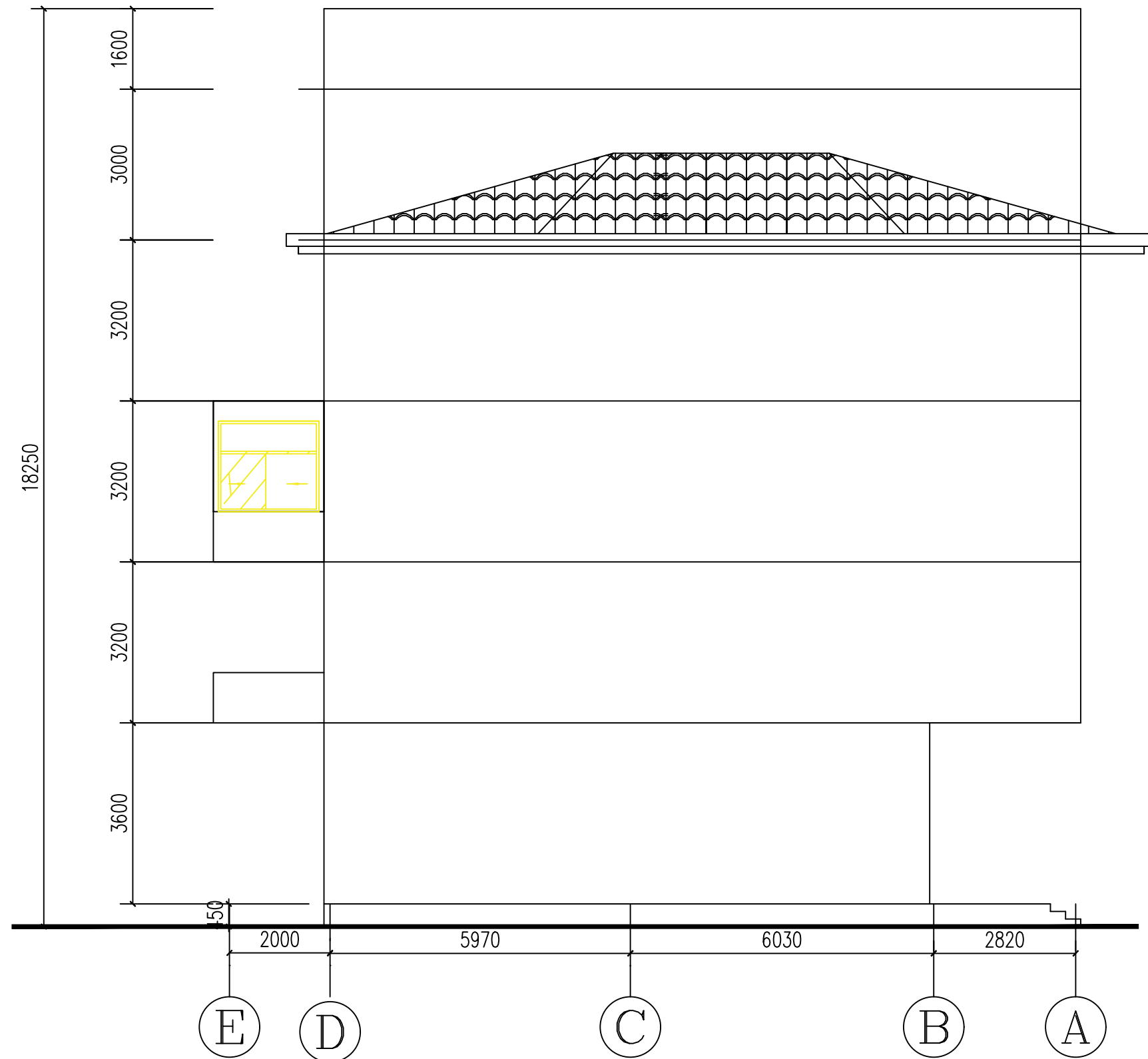
⑤—① 轴立面图 1:150
