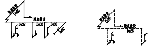
宿舍区卫生间大样图 1:100
