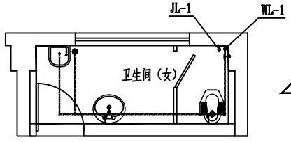
二~五层卫生间大样图 1:100
