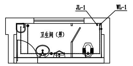
二~五层卫生间大样图 1:100
