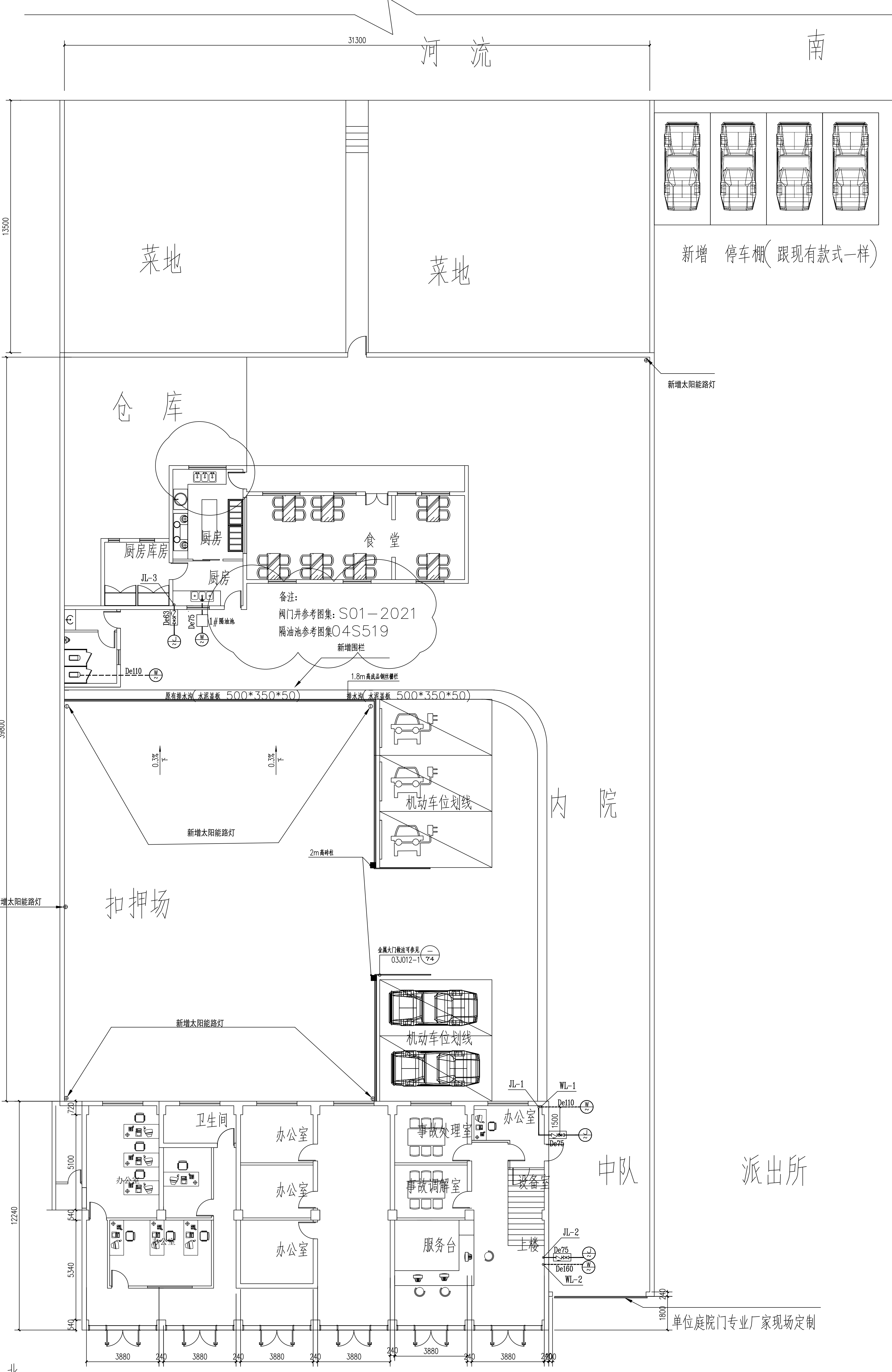
一层给排水平面图 1:100
