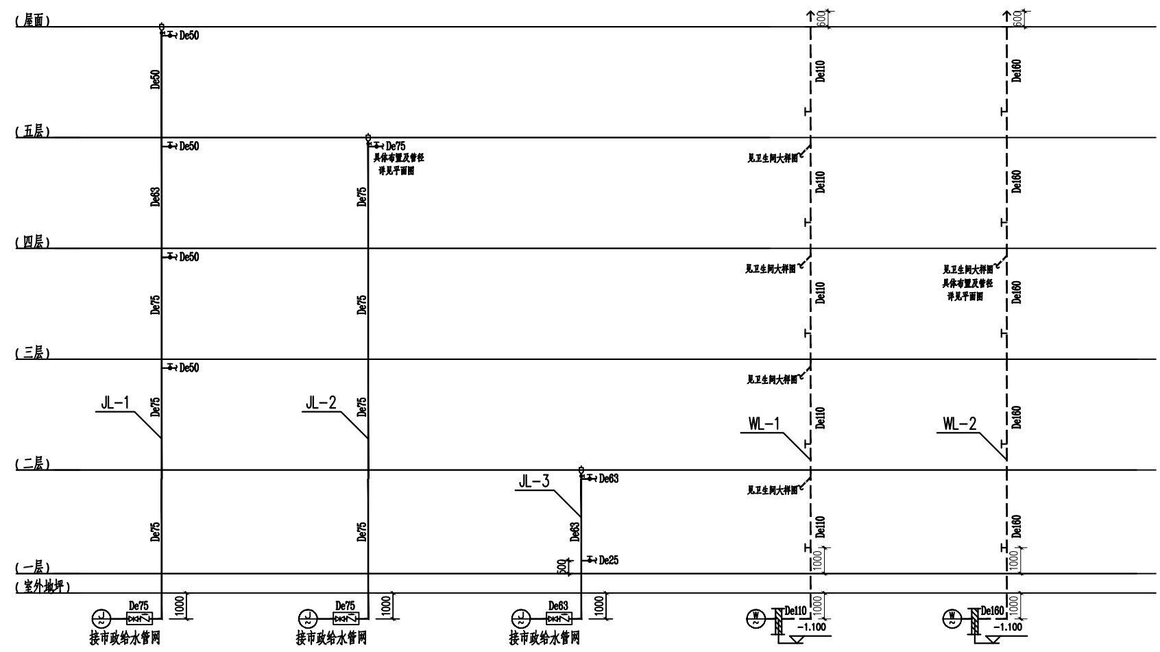
给排水系统图 1:100
