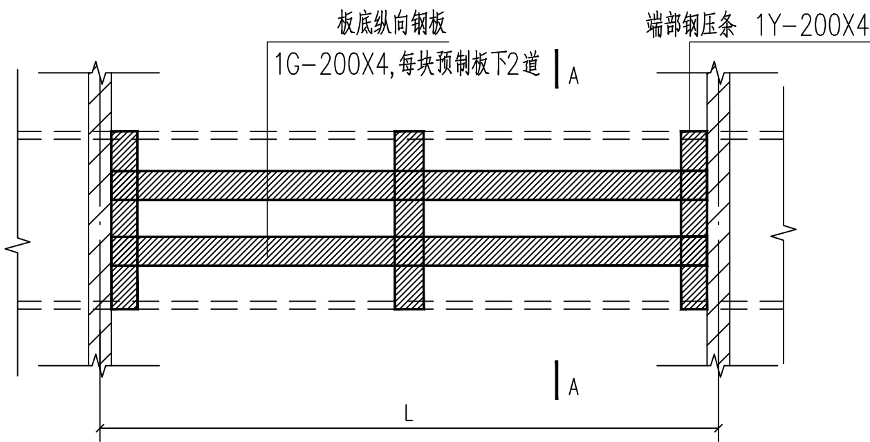
预制板板底贴钢板加固大样
