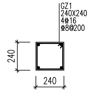
3-3 构造柱
