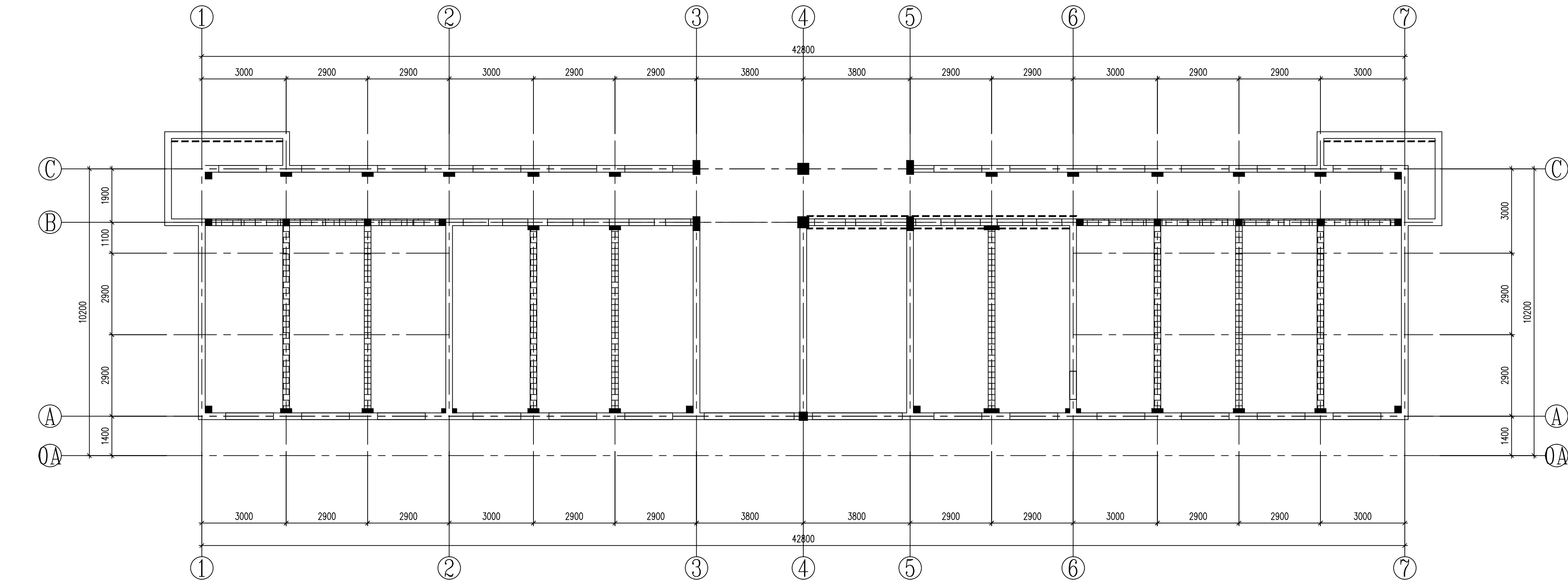
二层新增墙体平面布置图 1: 100
