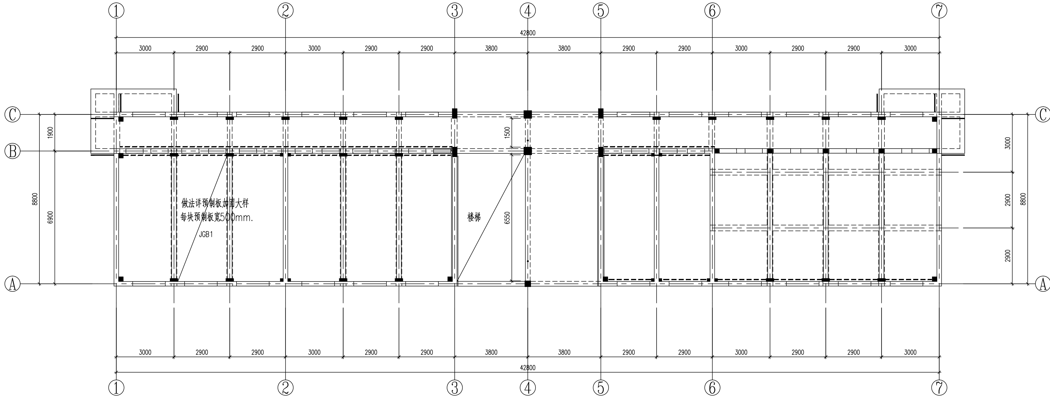
二层板底加固平面布置图 1:100
