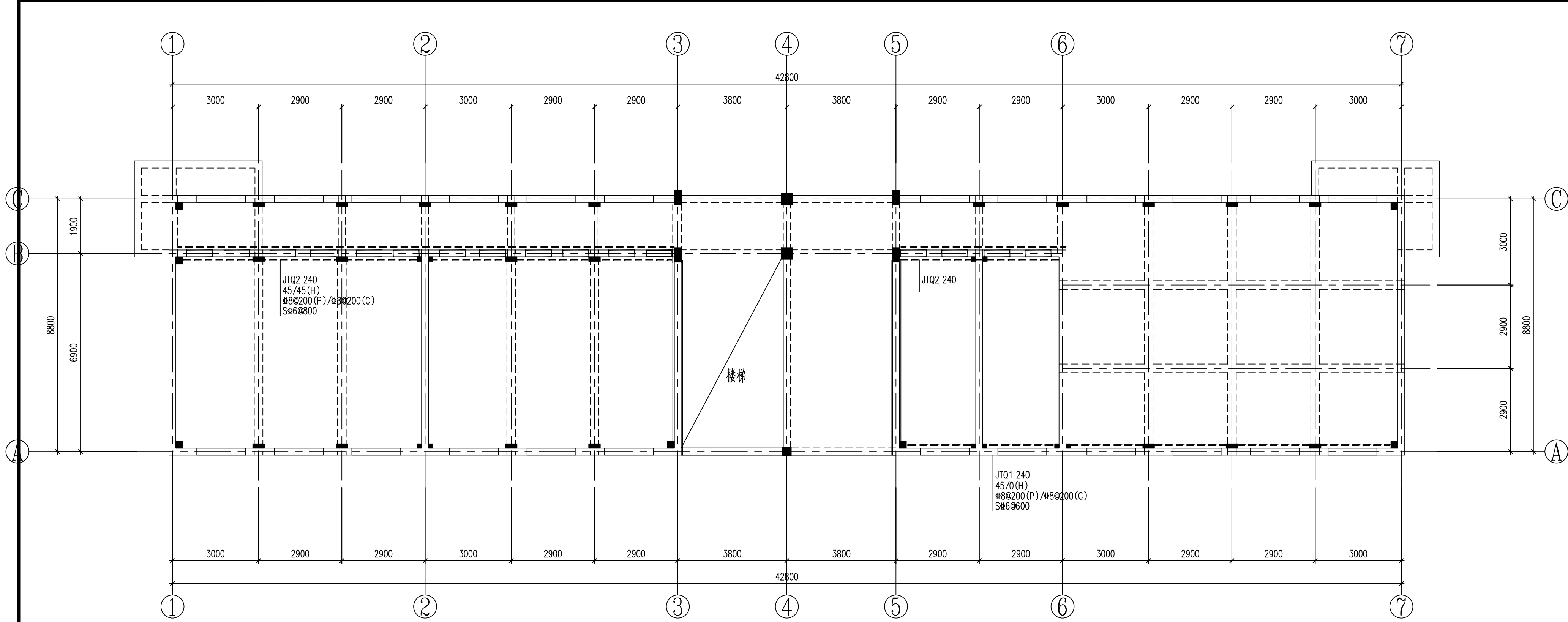
一层墙体加固平面布置图 1:100 基础顶~3.600m
