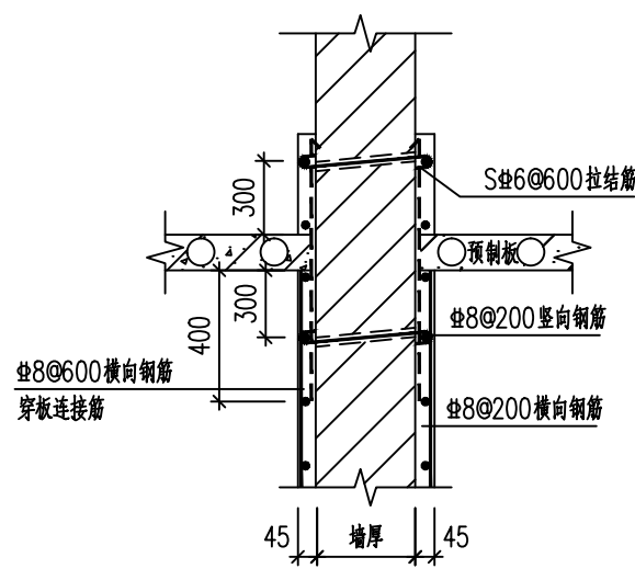
墙体楼板处做法(预制板) 1:20 采用高延性混凝土面层进行墙体加固。 上部墙不加固
