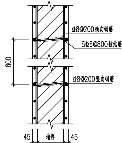
墙体双面加固大样 1:20 采用高延性混凝土面层进行墙体加固。
