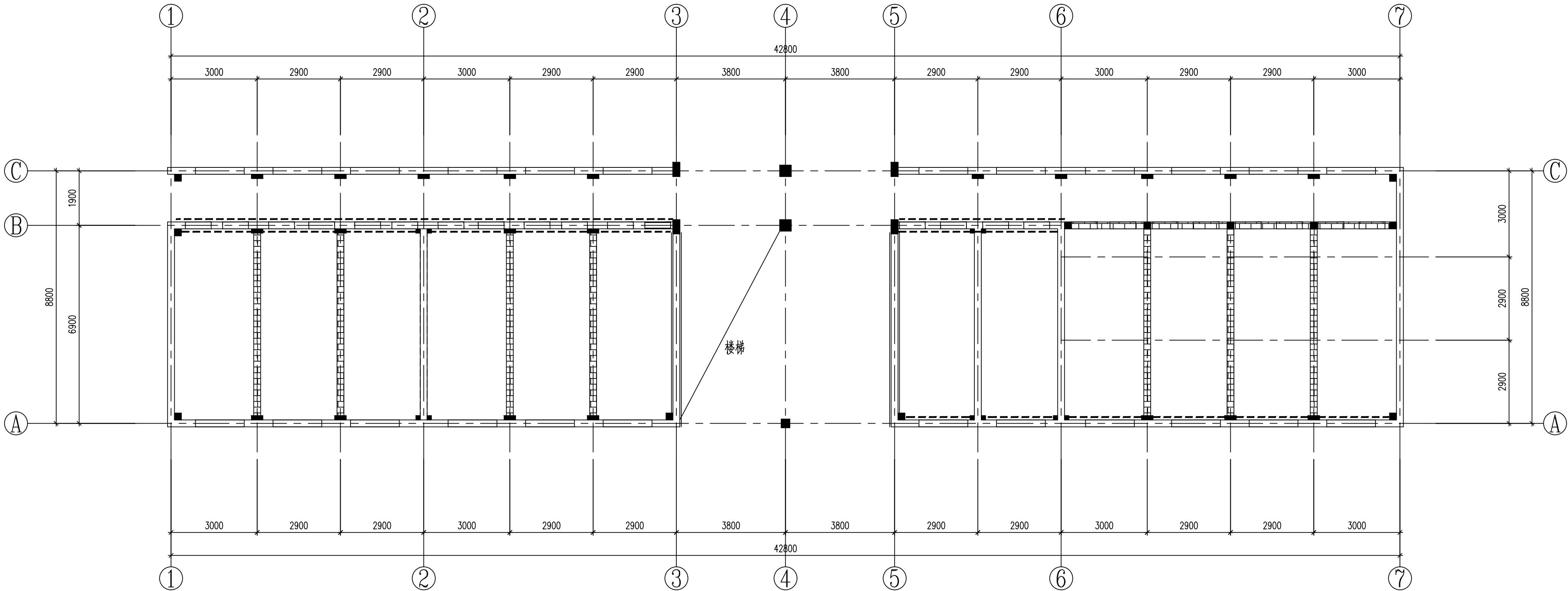
一层新增墙体平面布置图 1:100
