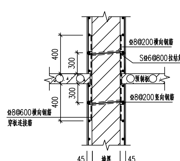
墙体楼板处做法(预制板) 1:20 采用高延性混凝土面层进行墙体加固。
