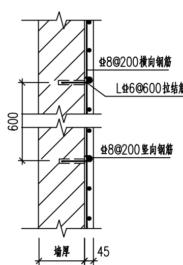
墙体单面加固大样 1:20 采用高延性混凝土面层进行墙体加固。
