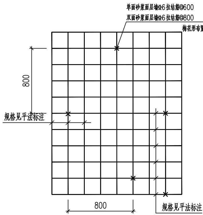
钢筋网及拉结筋示意图
