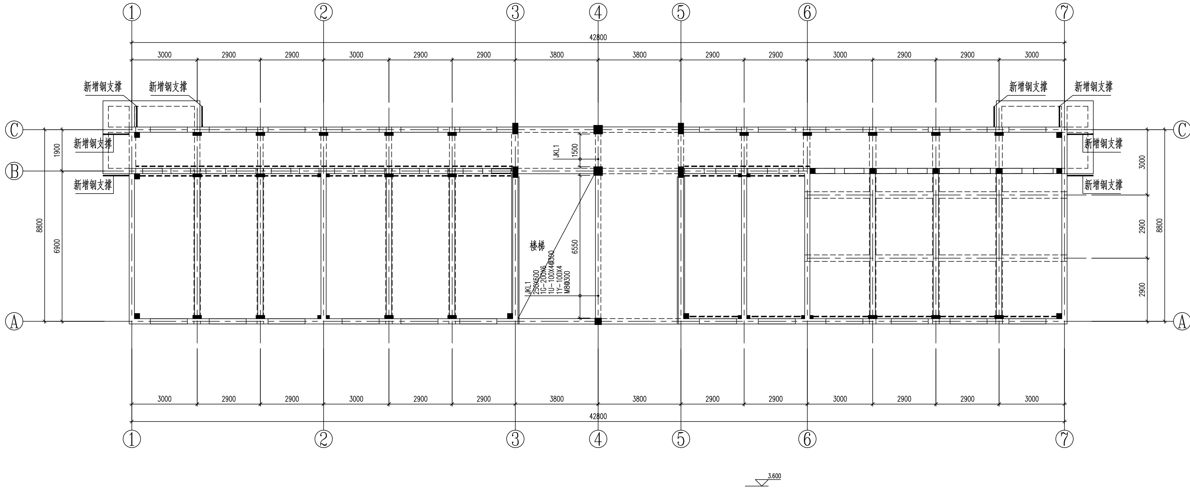
二层梁加固平面布置图 1:100
