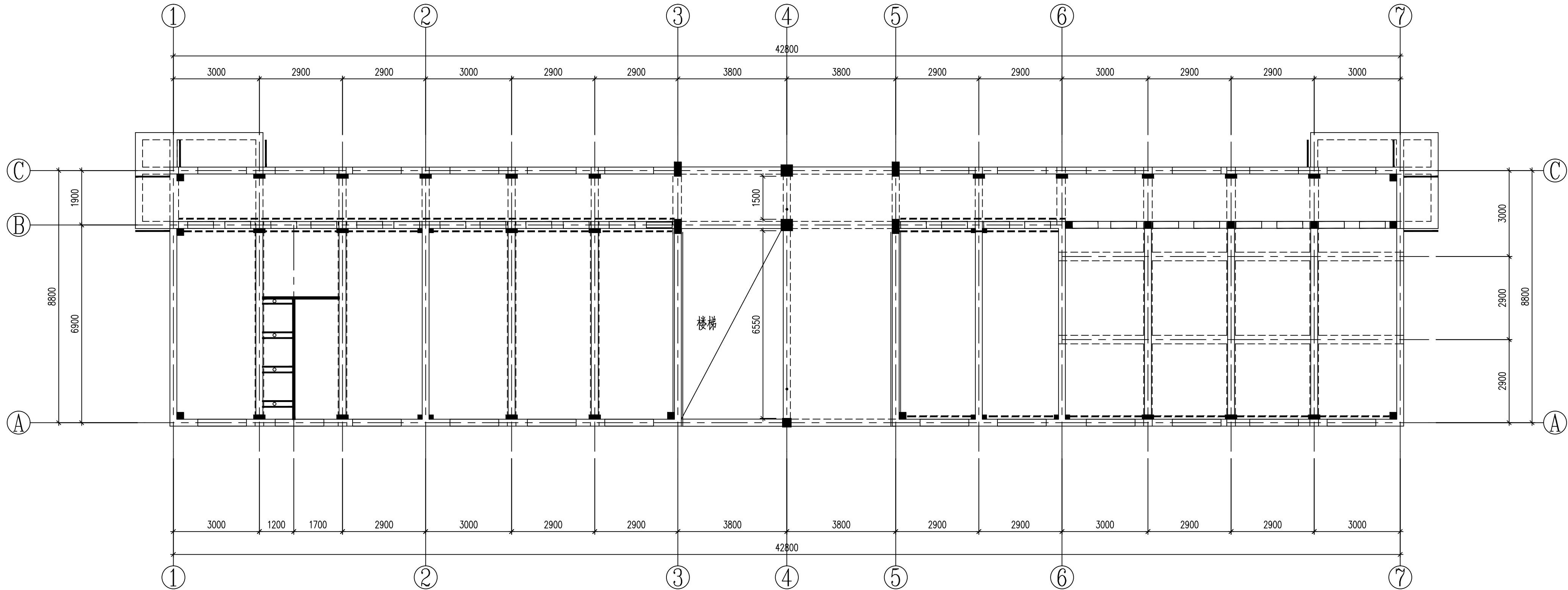
二层改造加固后结构平面布置图 1:100
