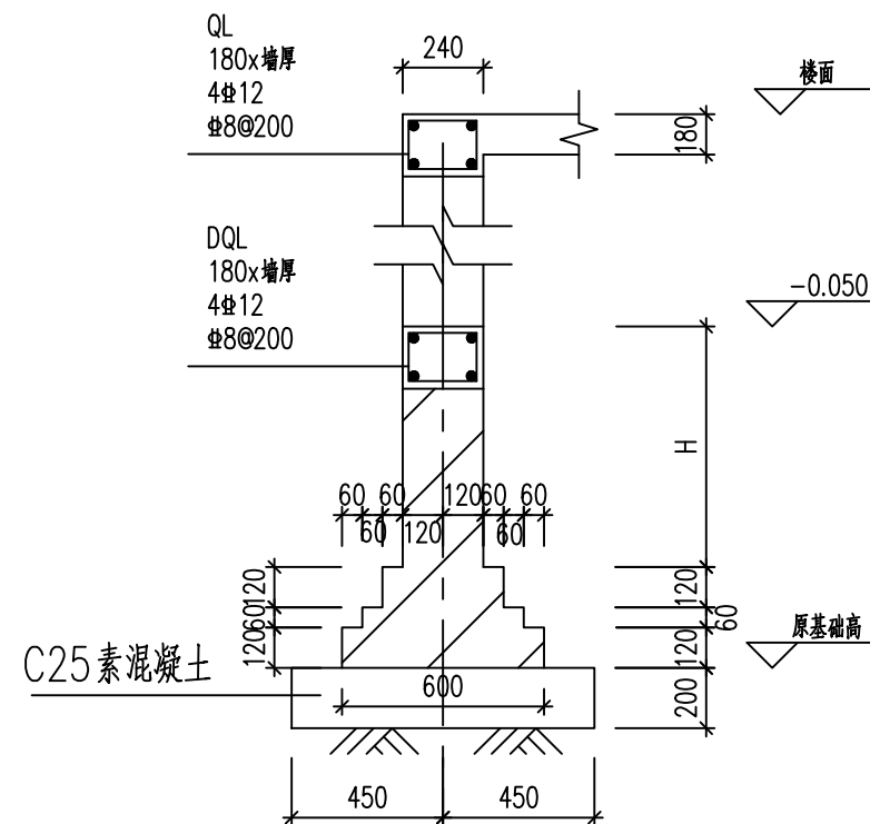
新增墙基础大样
