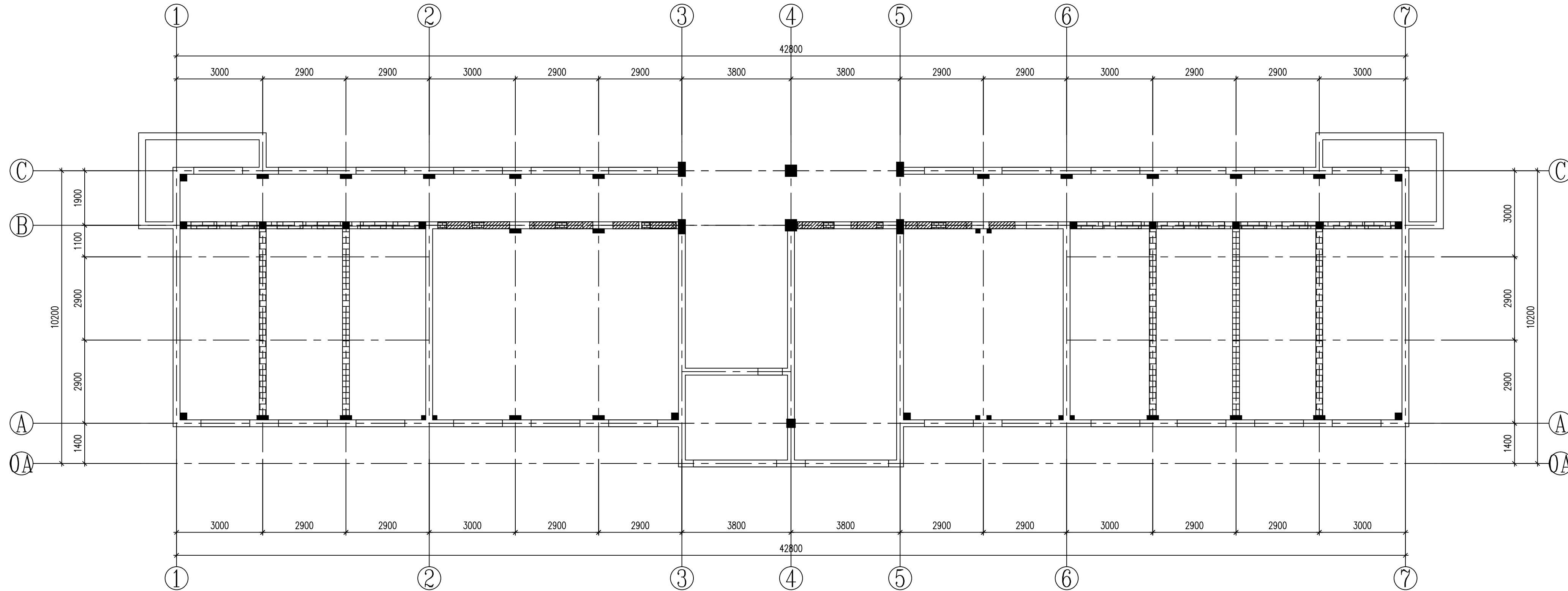
三层新增墙体布置图 1: 100
