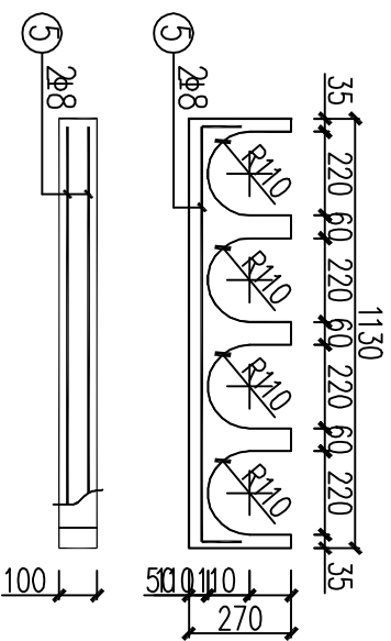
管枕C详图 1:20
