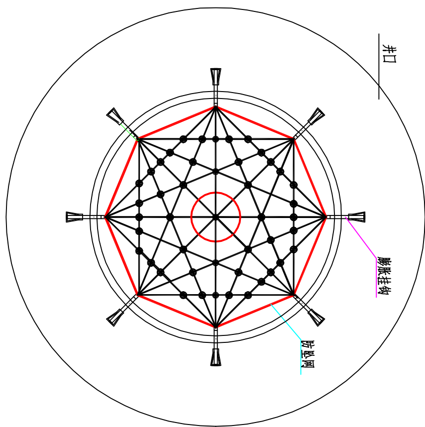
井筒防坠网安装平面图
