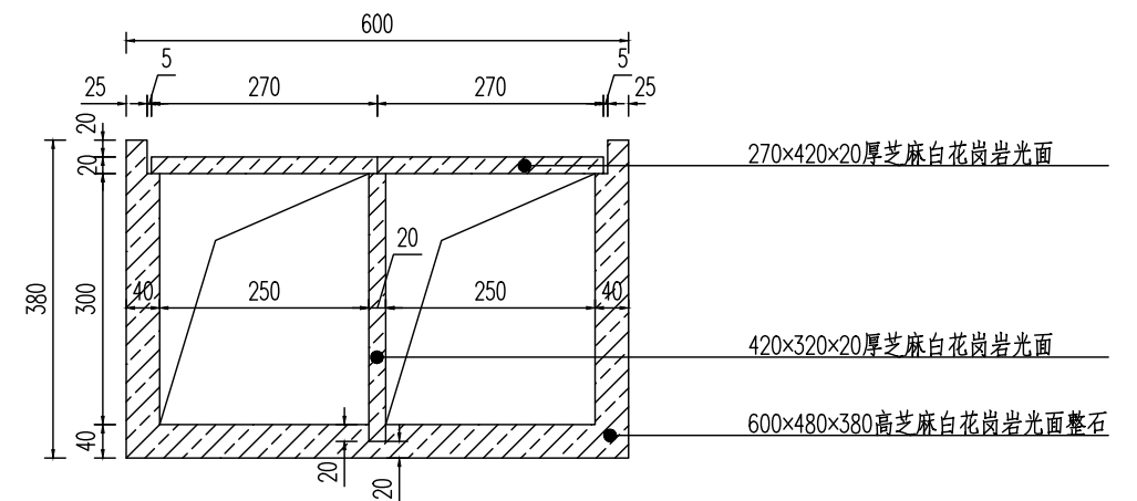
剖面图1 1:10
