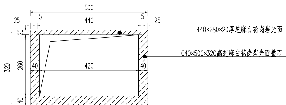
剖面图2 1:10
