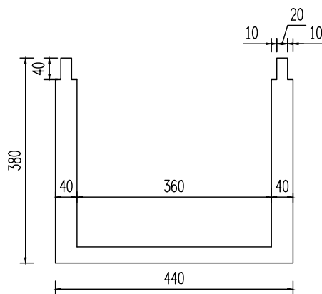
石箱剖面图
