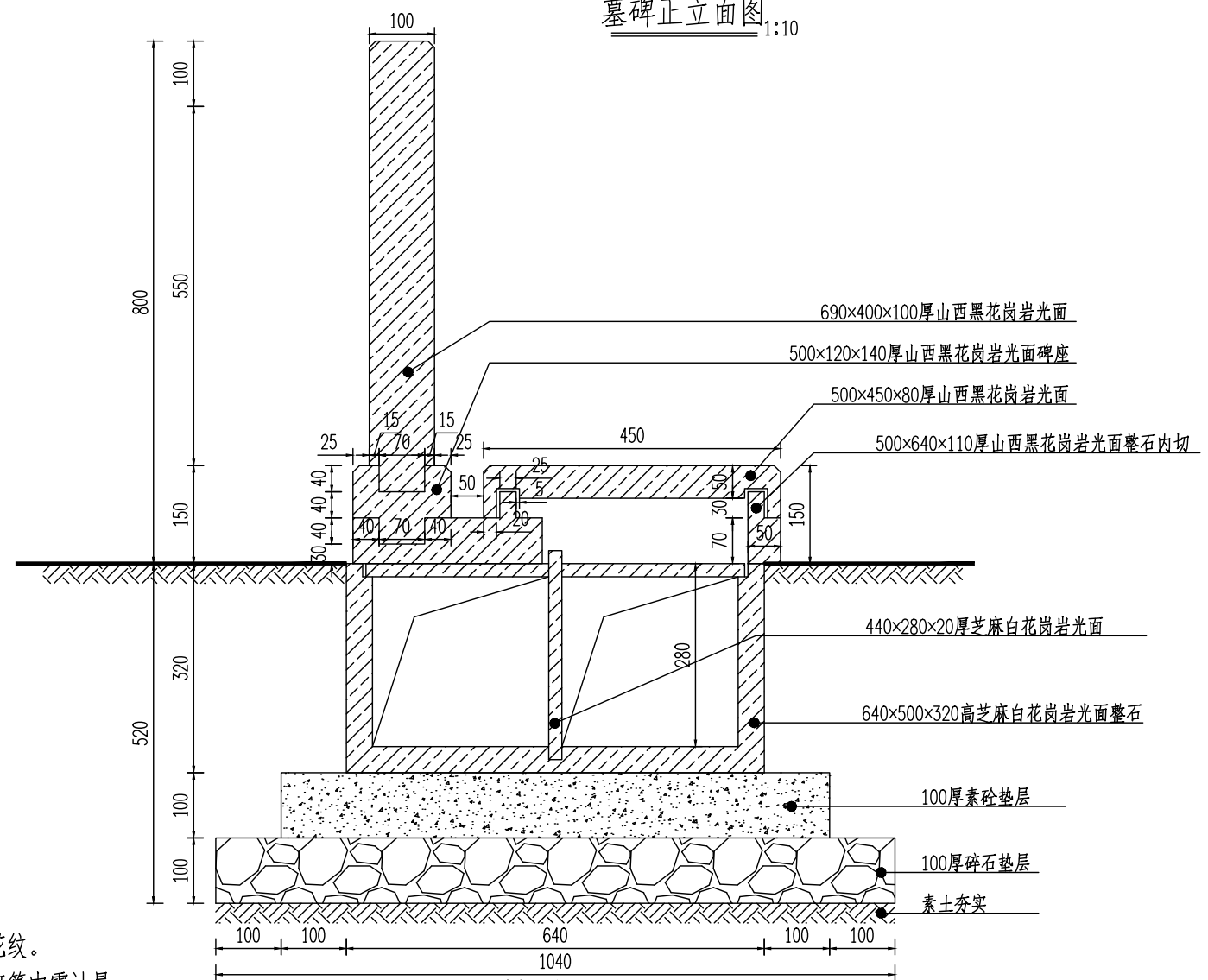
剖面图 1:10
