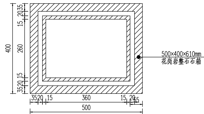
石箱俯视图 1:10
