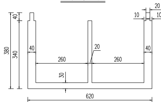
石箱剖面图
