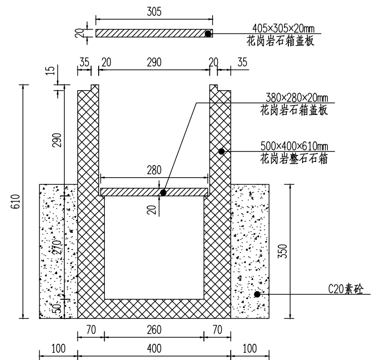
石箱侧视图 1:10
