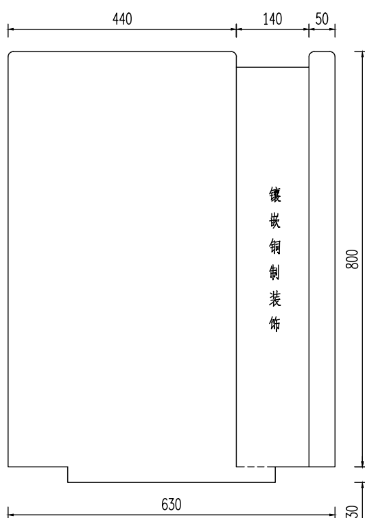
石碑平面图
