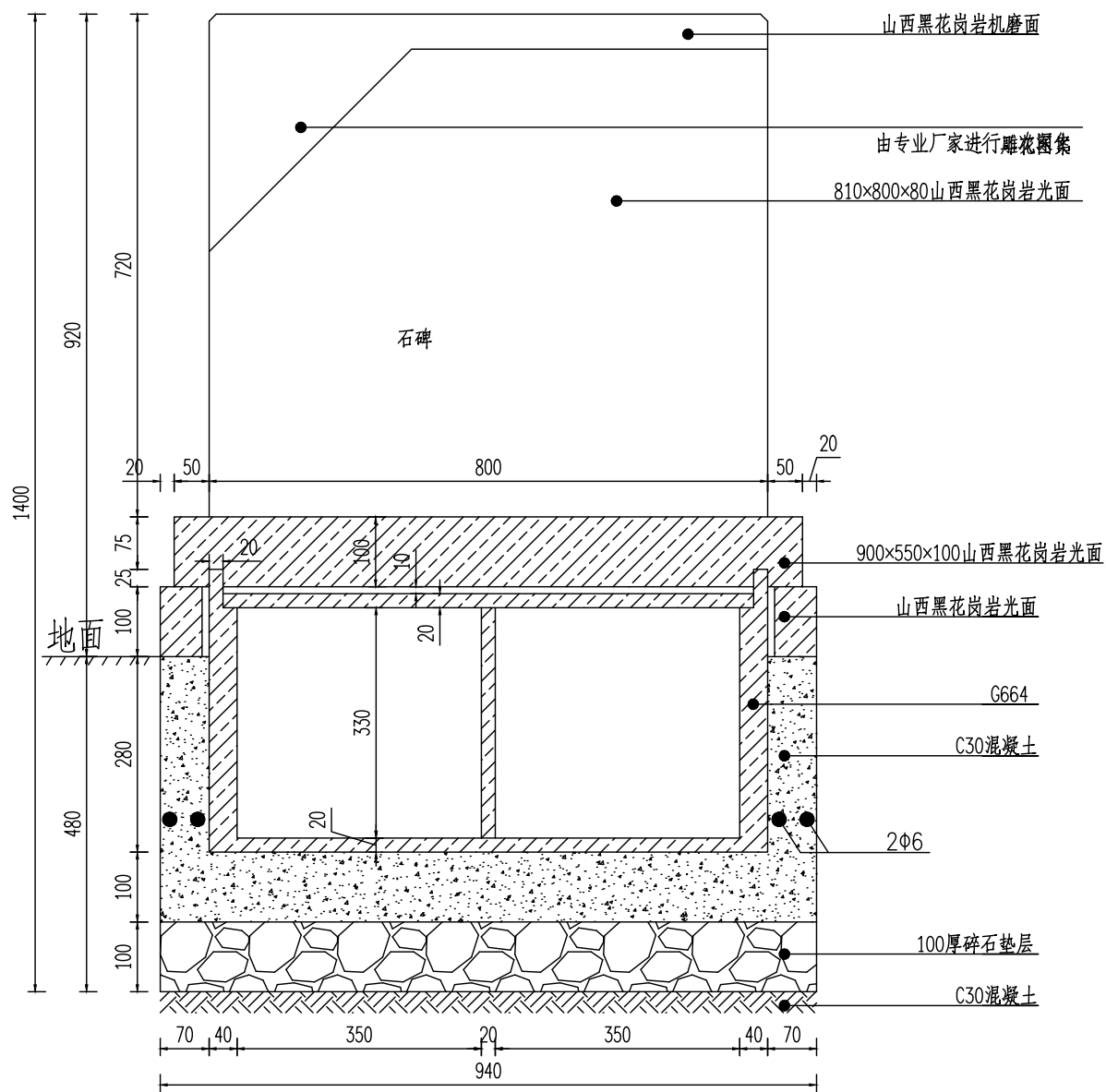
剖面图 1:10
