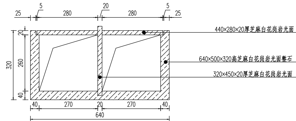
剖面图1 1:10
