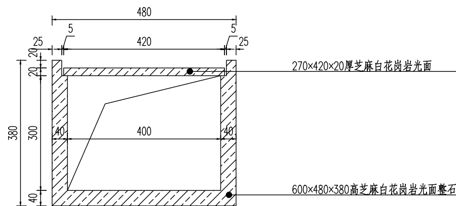
剖面图2 1:10
