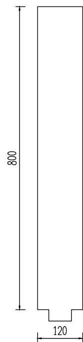
石碑侧面图
