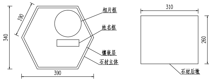
石盖平面图
