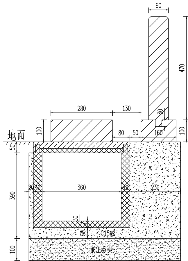
整体剖面图
