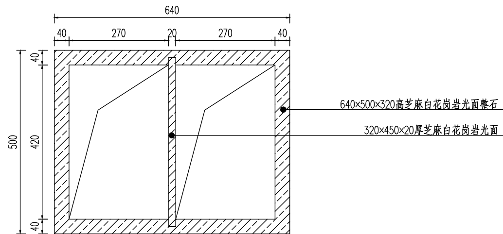
地宫截面图 1:10
