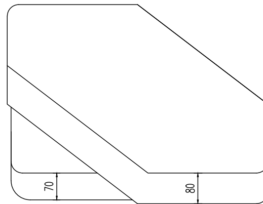
石盖侧面图
