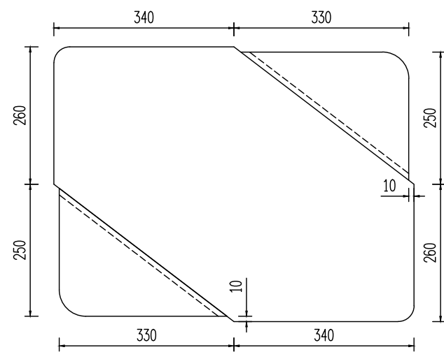
石盖平面图
