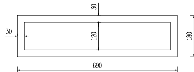
底座平面图
