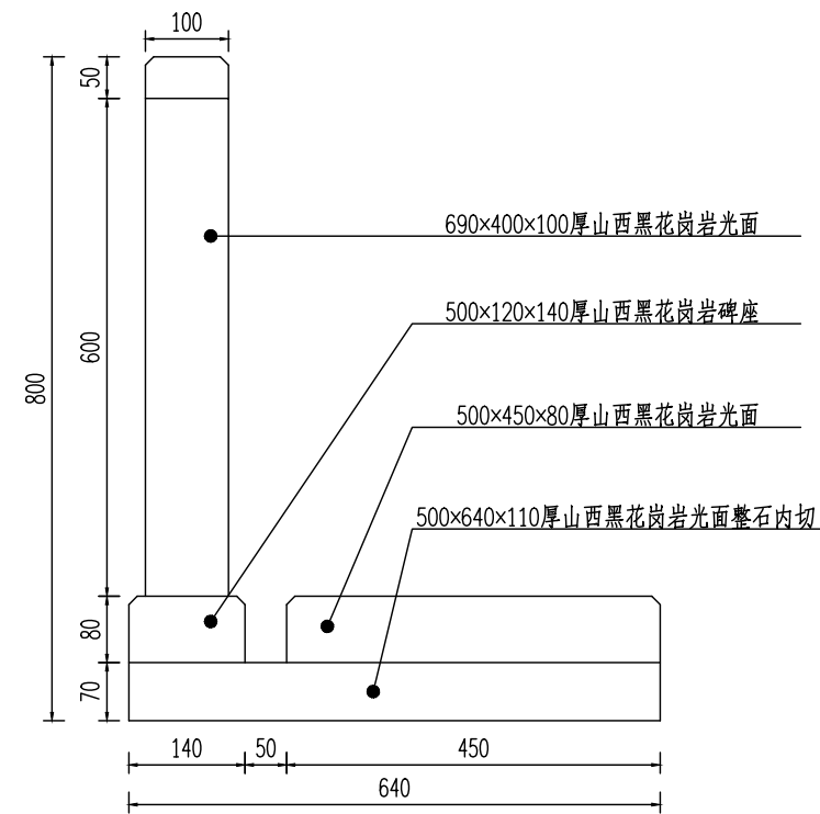
墓碑侧立面图 1:10
