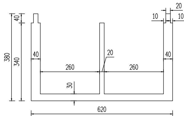
石箱剖面图
