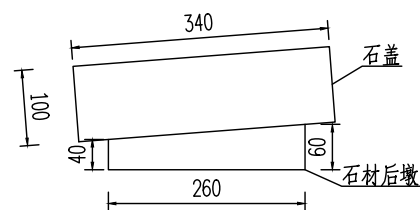
石盖侧面图
