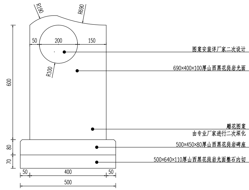
墓碑正立面图 1:10
