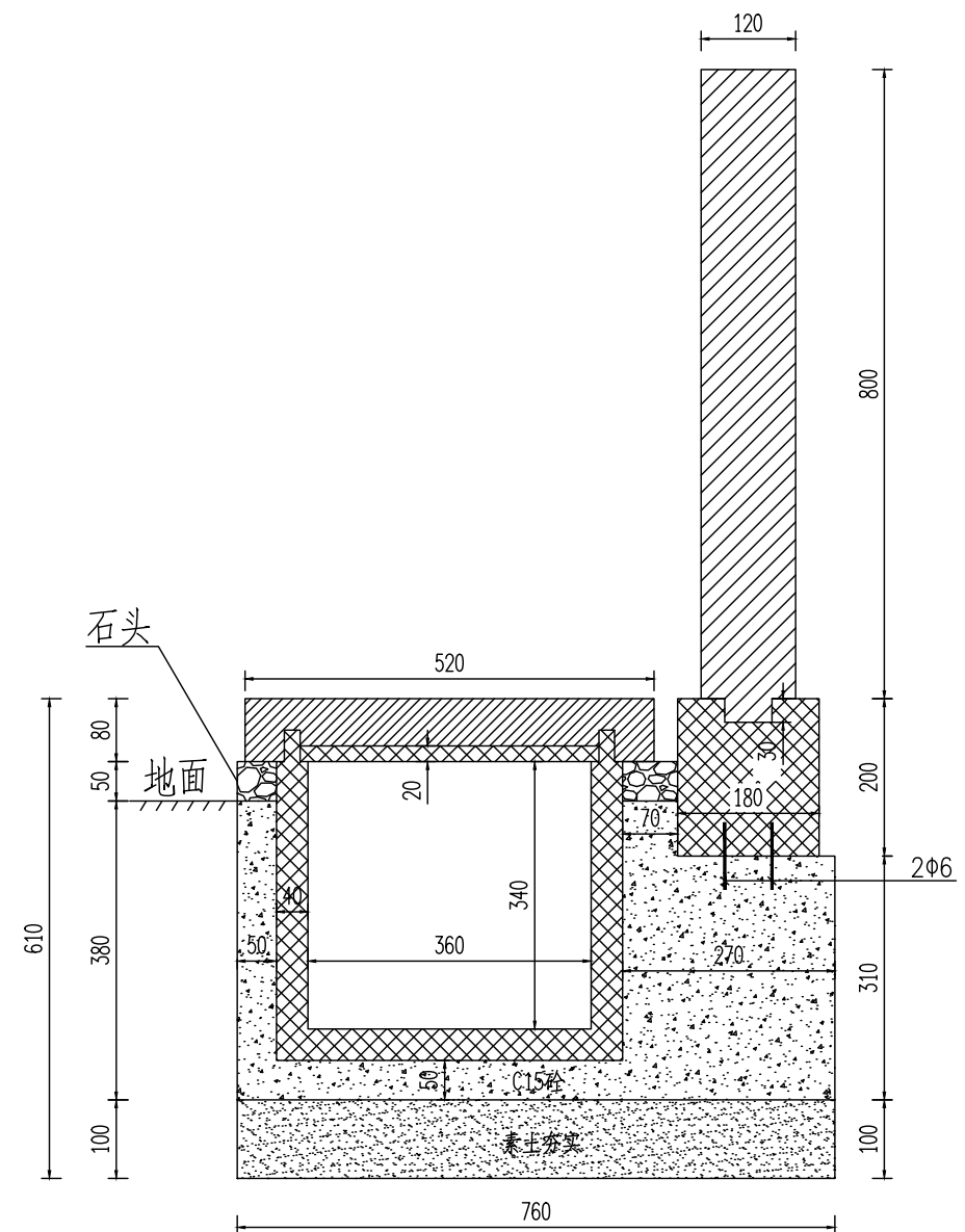
整体剖面图
