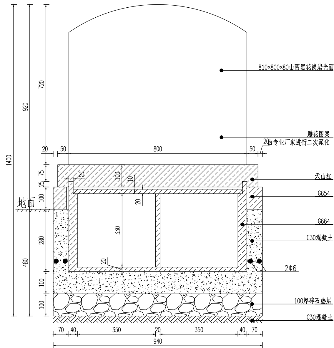
剖面图 1:10
