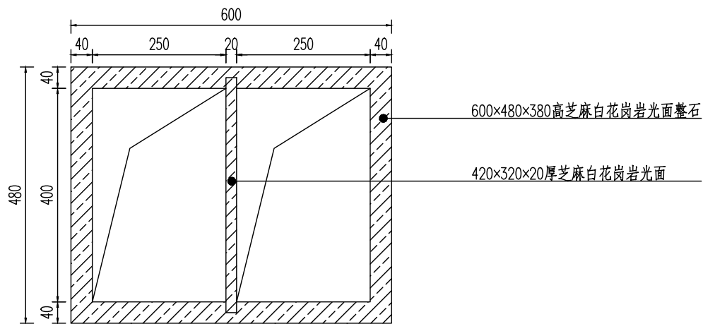
地宫截面图 1:10
