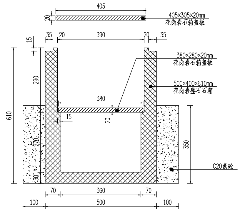
石箱正视图 1:10
