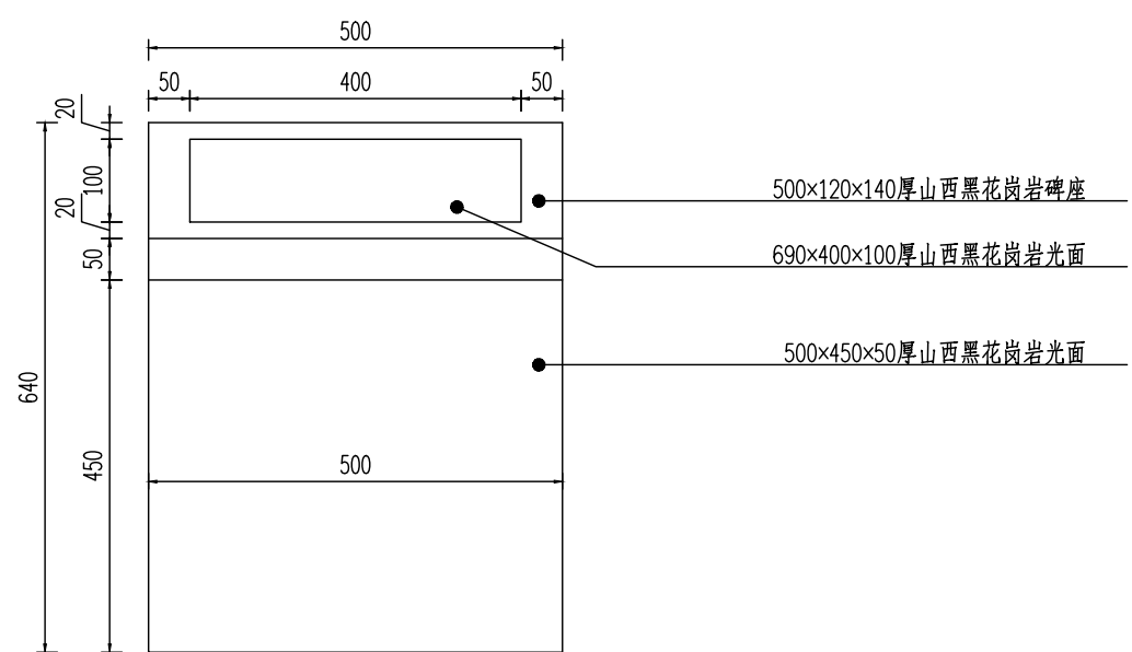
墓碑平面图 1:10
