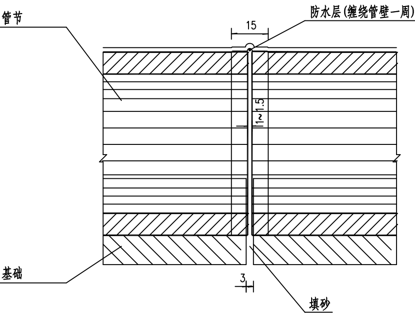
沉降缝
