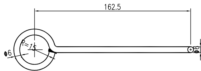
固定钩
