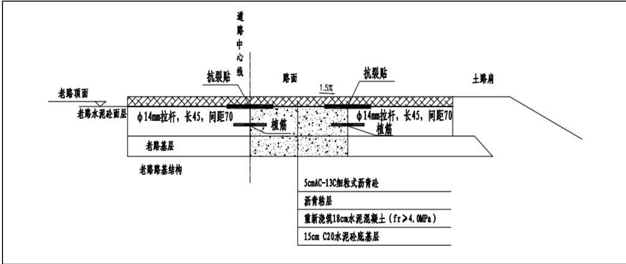
图7-1 K0+510～K0+735段病害处理结构图
