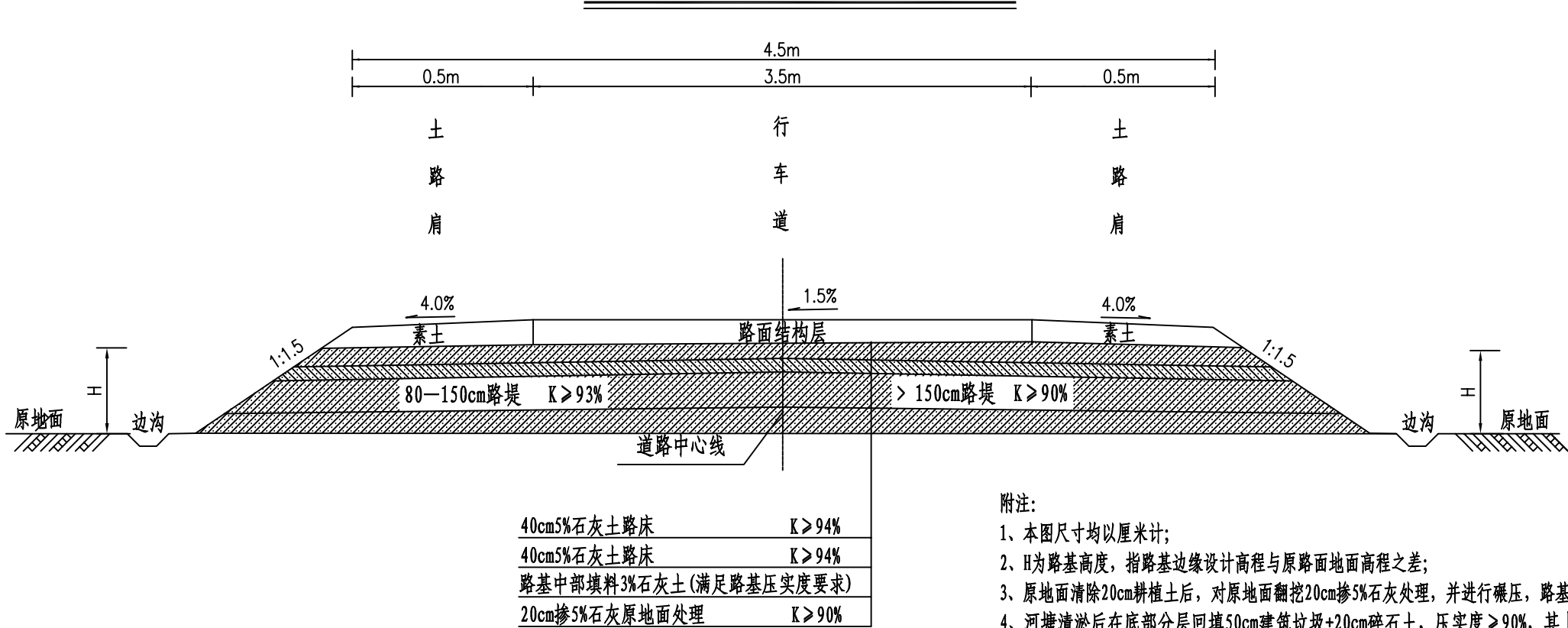
路基一般设计图二（H > 0.84m）
