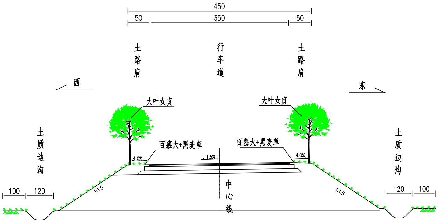
绿化美化横断面图
