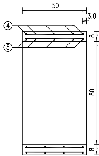
0.5米正管节纵断面
