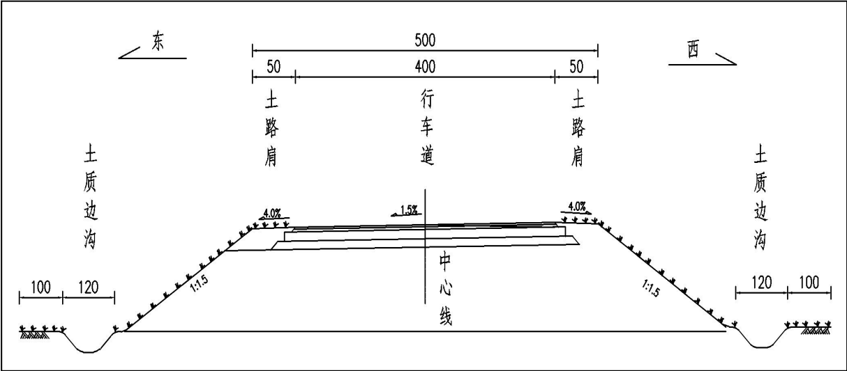
图3-2 K0+510～K0+735段路基标准横断面图
