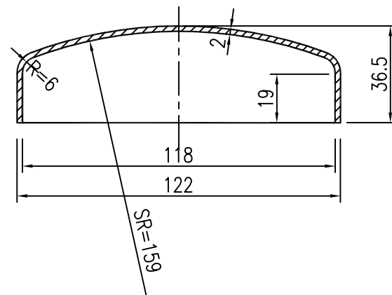
帽 盖
