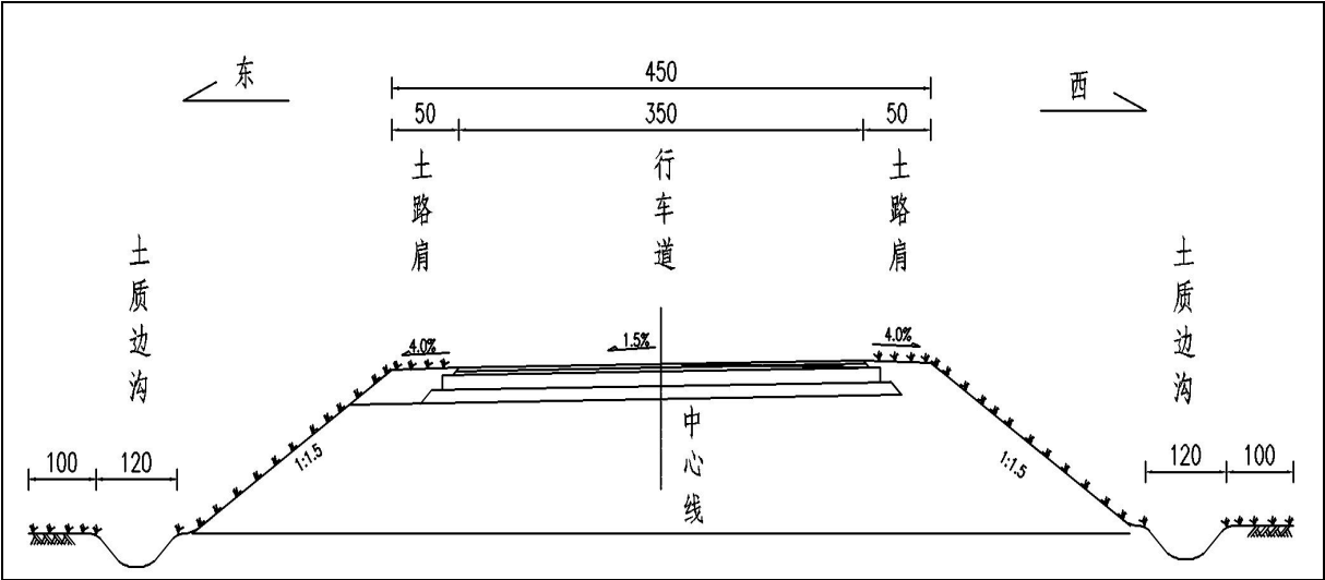
图3-1 K0+000～K0+510段及K0+735～K1+037.410段路基标准横断面图
