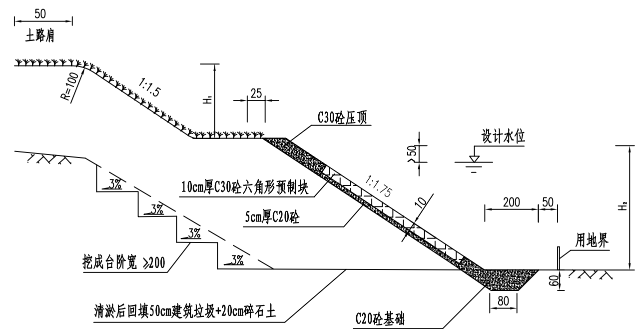
沿河水塘路段防护工程图
