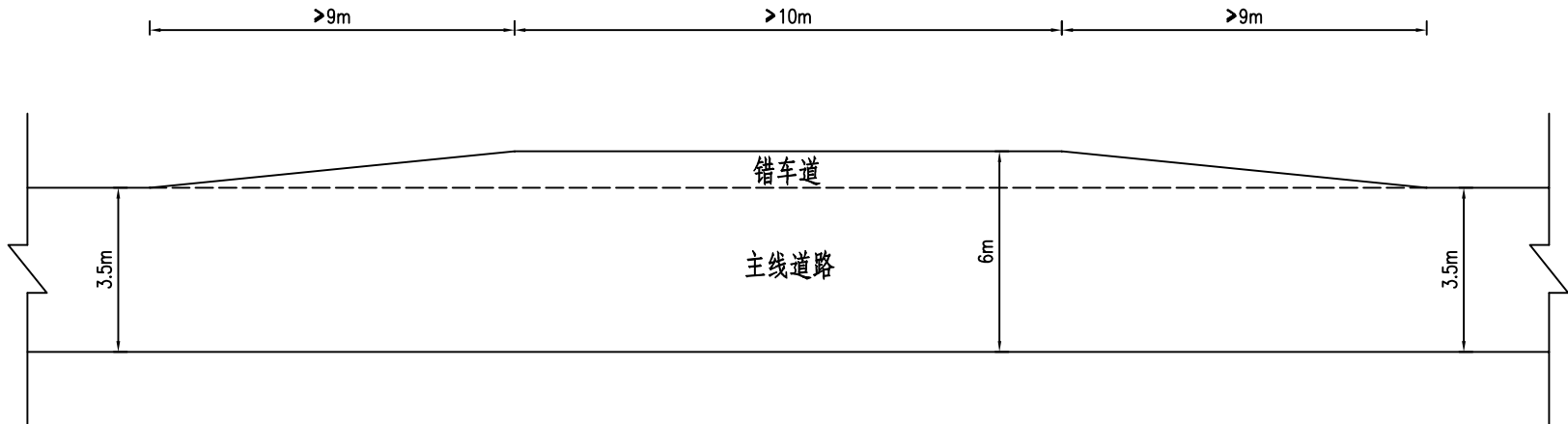
错车道工程数量表
