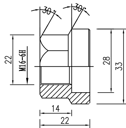
防盗压紧螺母A
