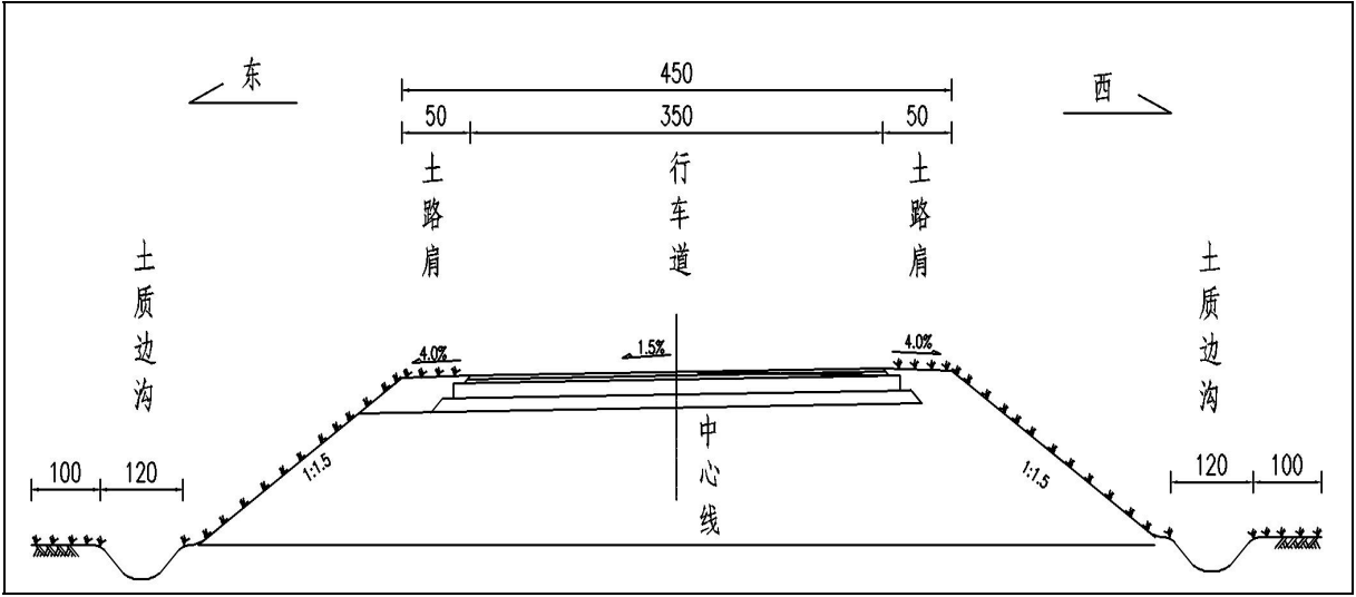
图 3-1 K0+000～K0+510 及 K0+735～K1+037.410 段路基标准横断面图
