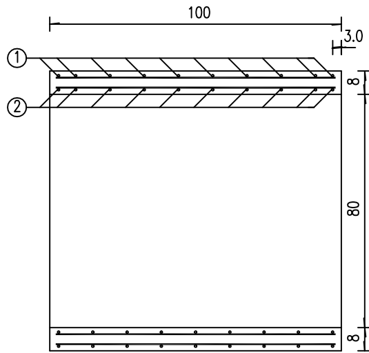
1米正管节纵断面
