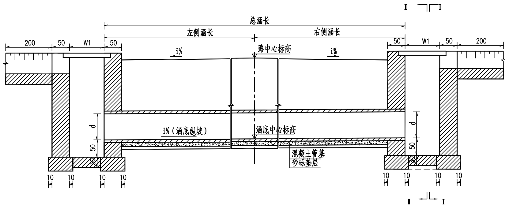
立面
