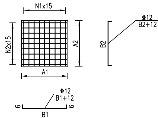
尺寸表 (cm)
