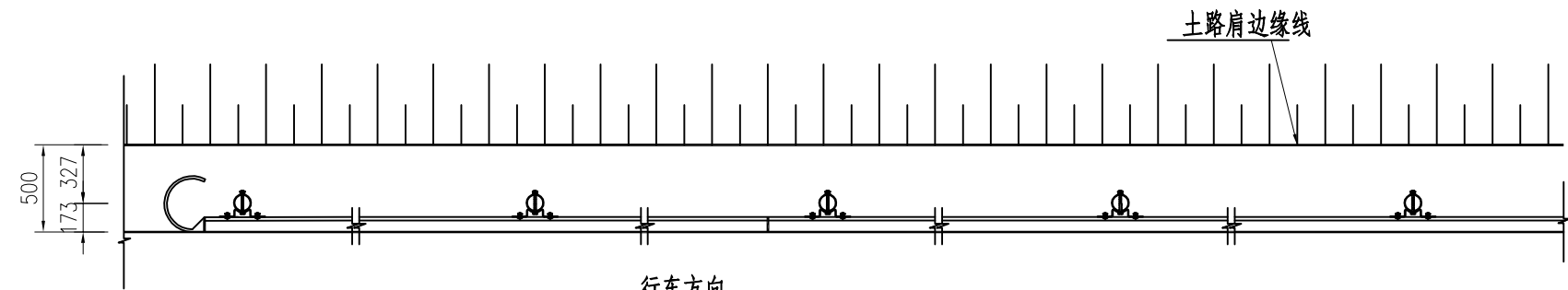
C级护栏上、下游端头平面图 1: 40
