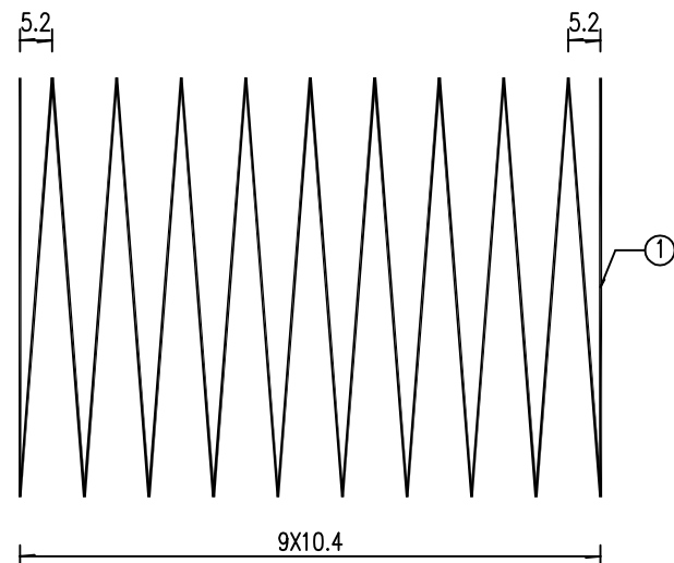
Φ8 96 ③
