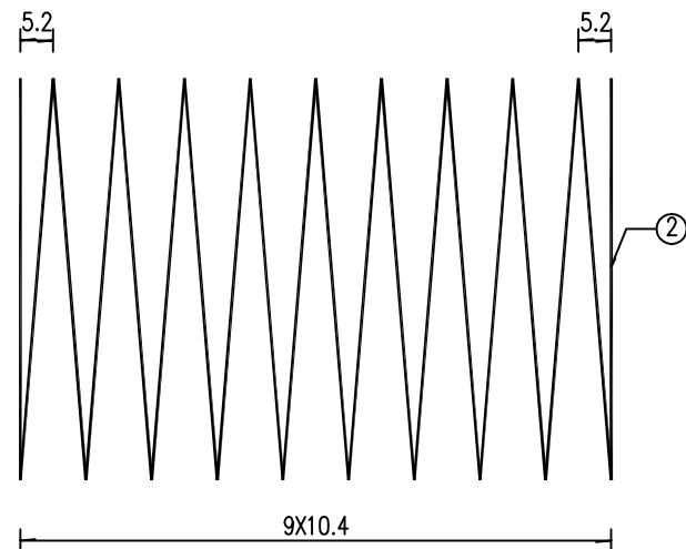
内圈螺旋形主钢筋
