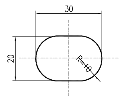
C向 1:1
