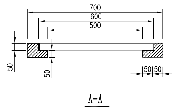
井框图
