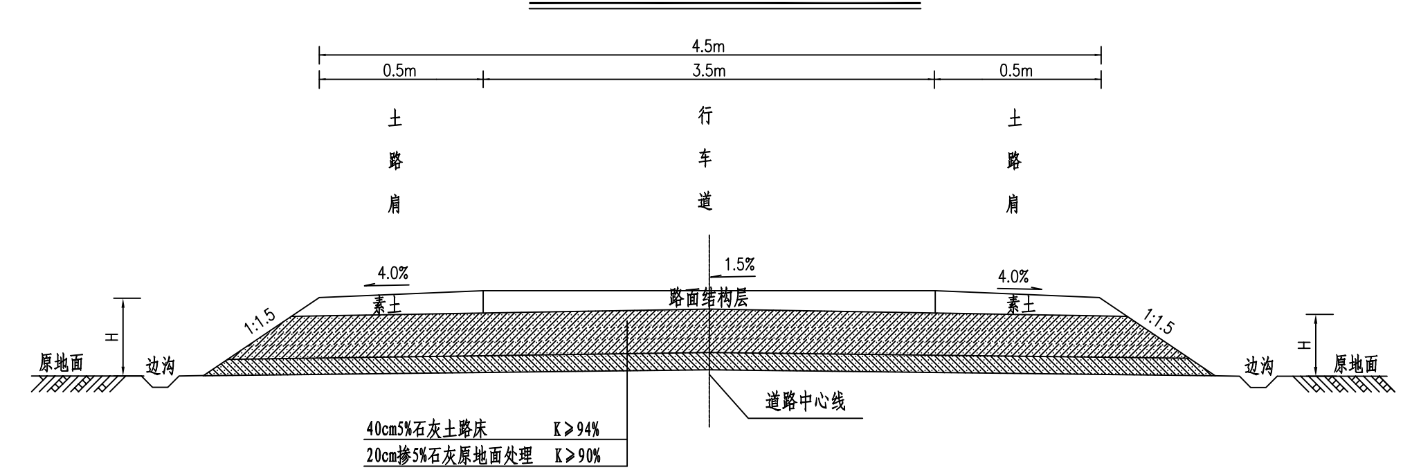
路基一般设计图一（H≤0.84m）
