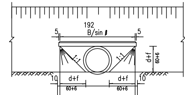
正涵身尺寸表
