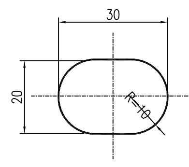
B向 1:1
