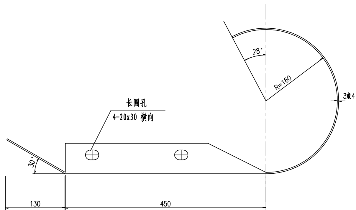
平面 1:5
