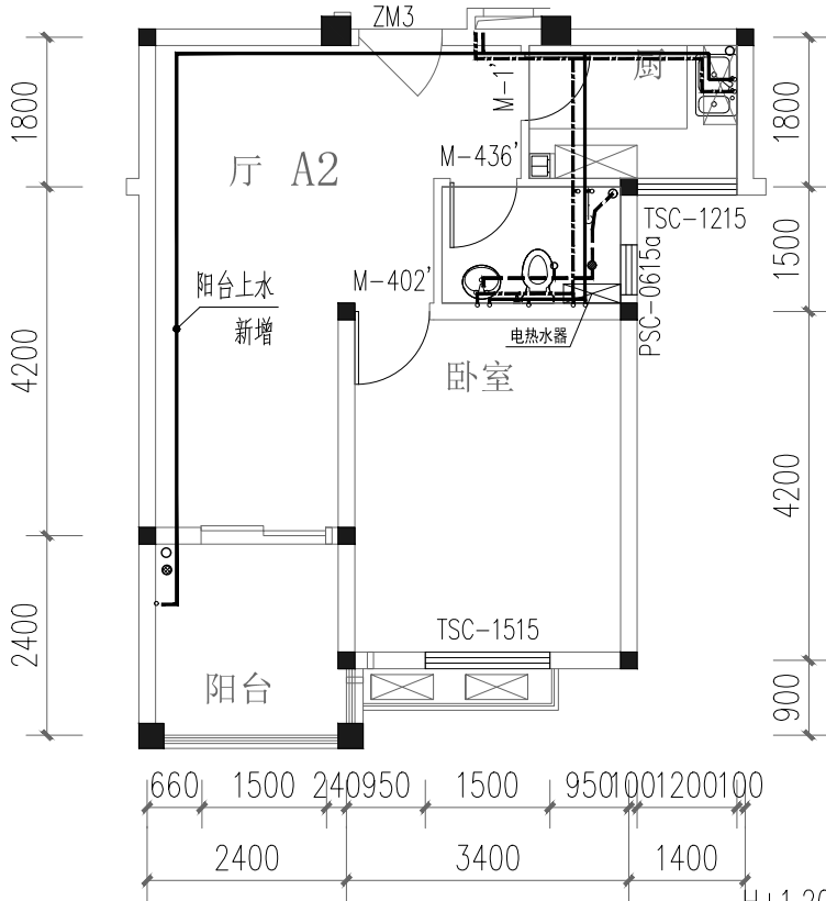
户型冷热水布置图 1:100
