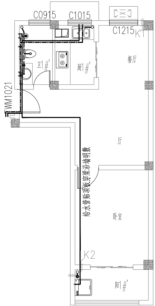
户型冷热水布置图 1:100
