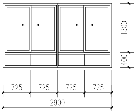
C2917 1:50
