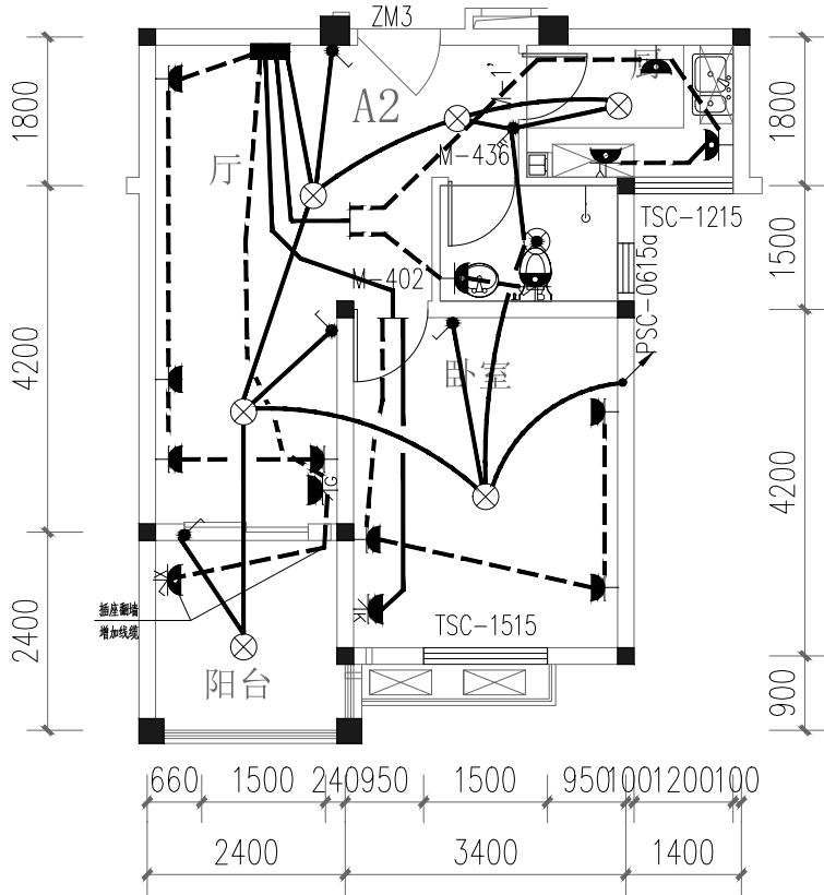
户型强电布置示意图 1:100
