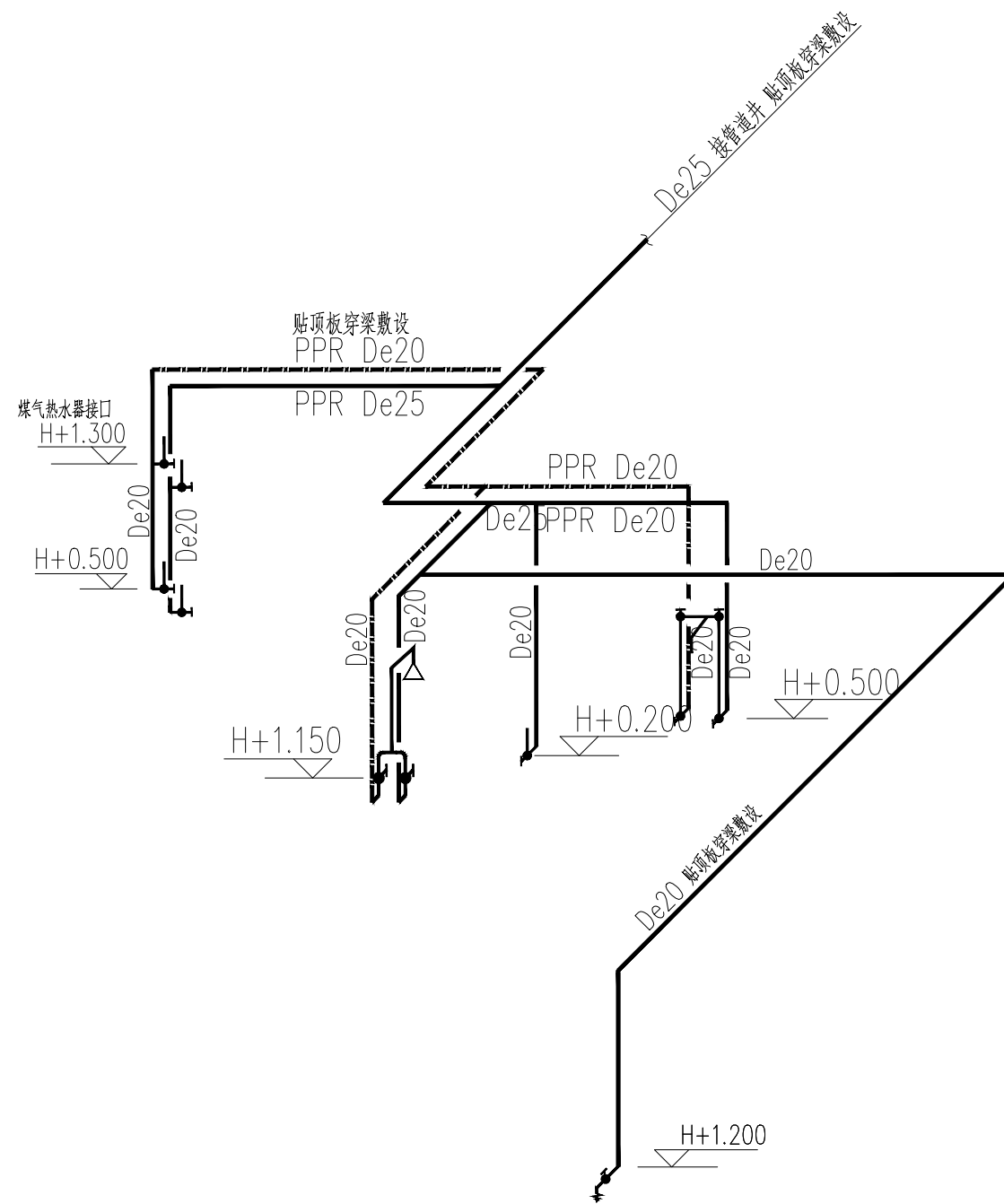
户型厨、卫给水支管详图
