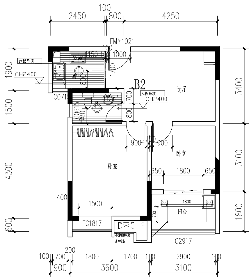
户型平面图 1:100
