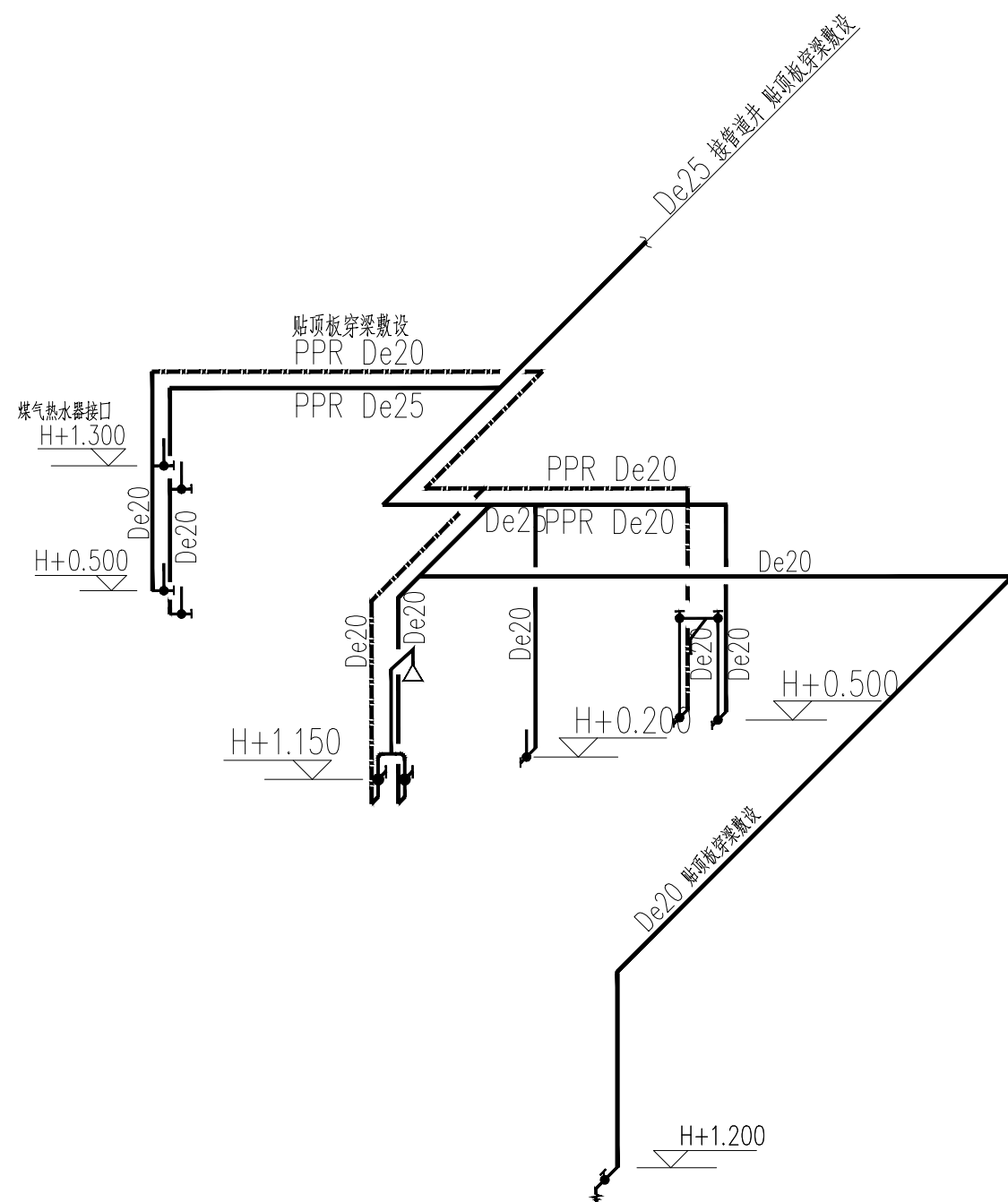
户型厨、卫给水支管详图
