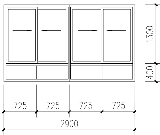
C2917 1:50
