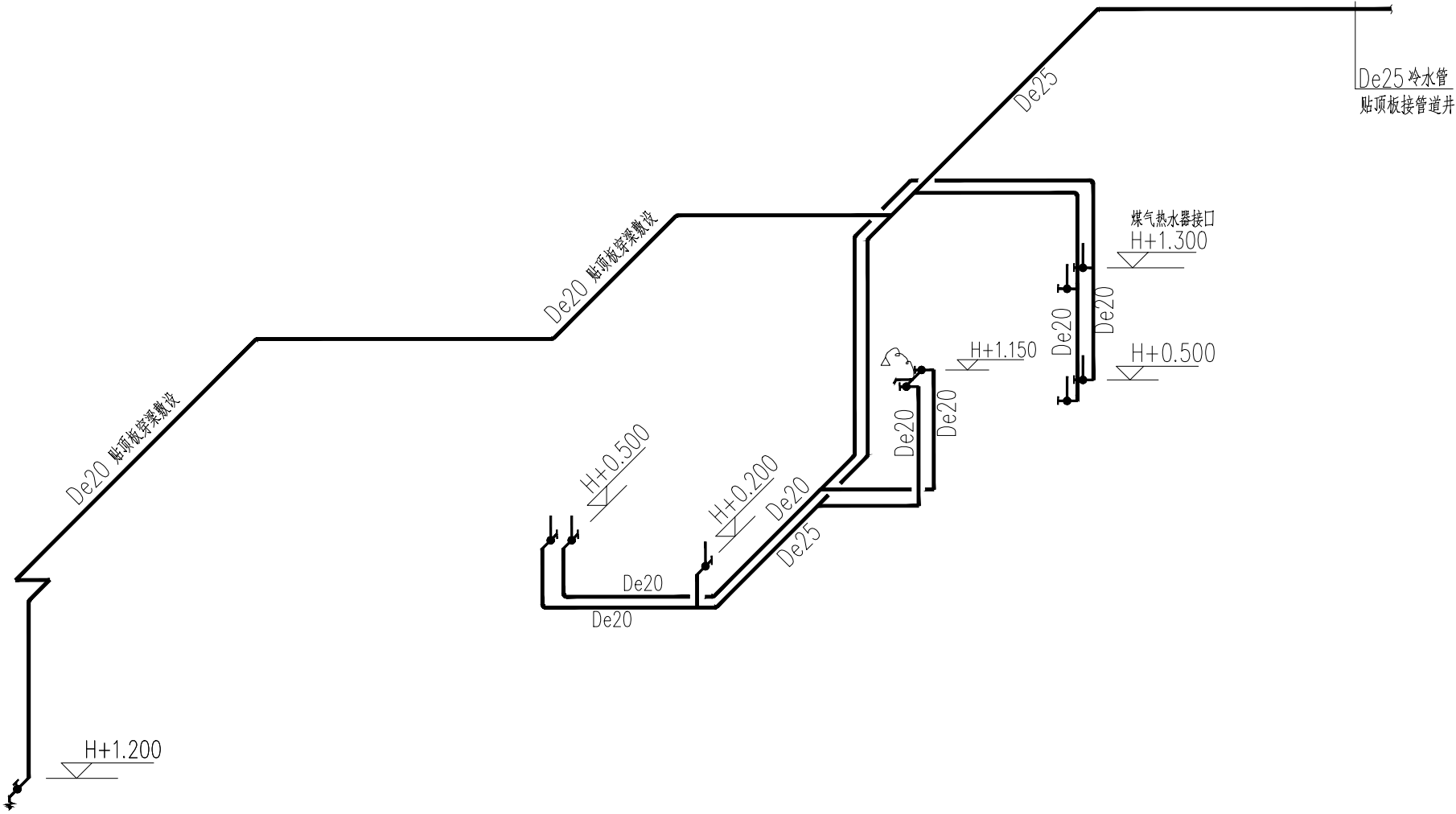
户型厨、卫给水管详图 1:50 注：冷热水管已安装到位
