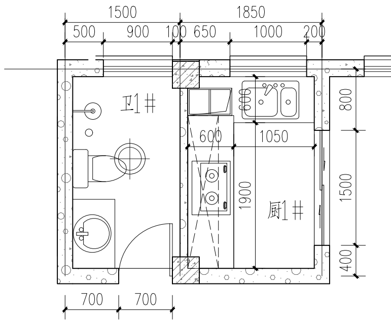
厨、卫平面详图 1:50
