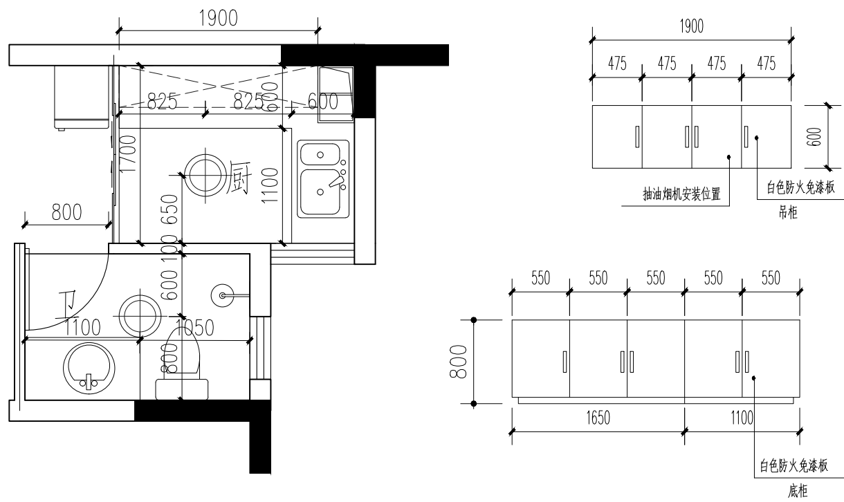
厨、卫平面详图 1:50
