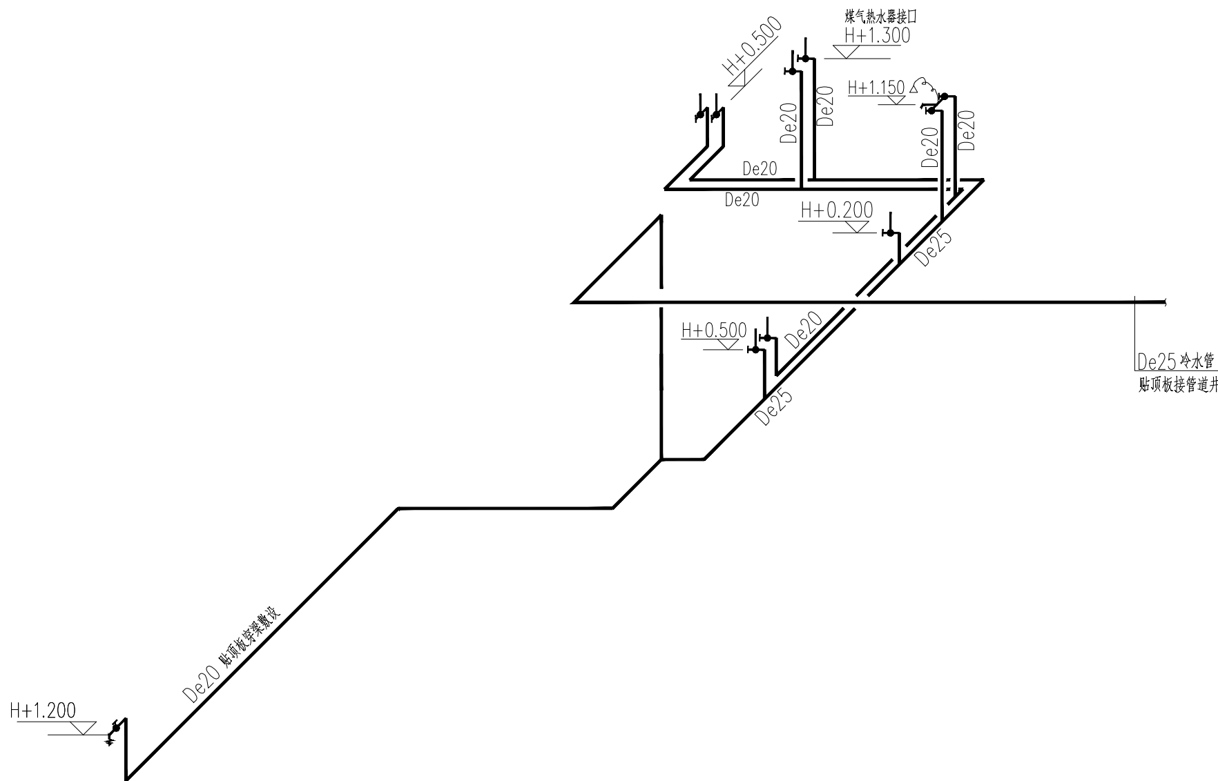
户型厨、卫给水支管详图 1:50
