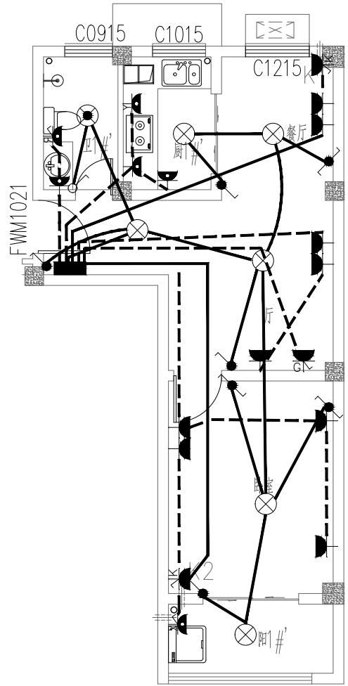
户型强电布置示意图 1:100
