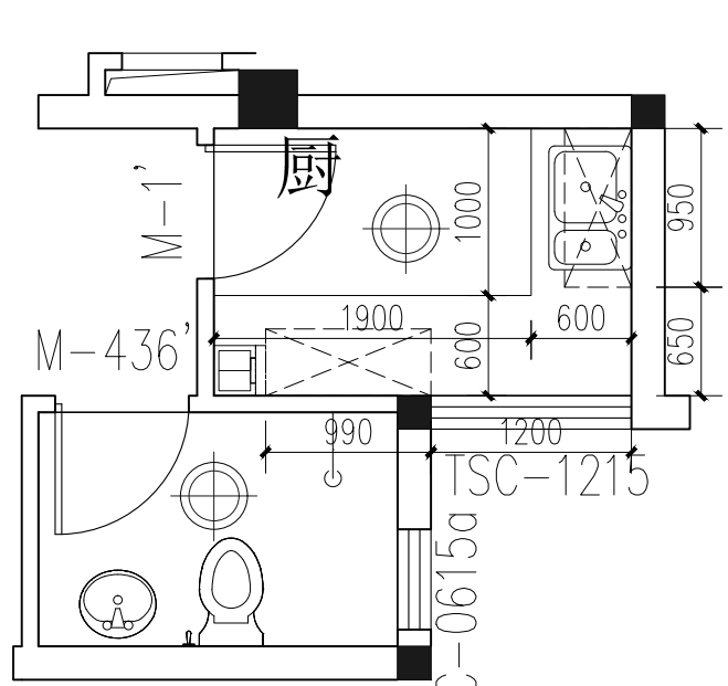
厨、卫平面详图 1:50
