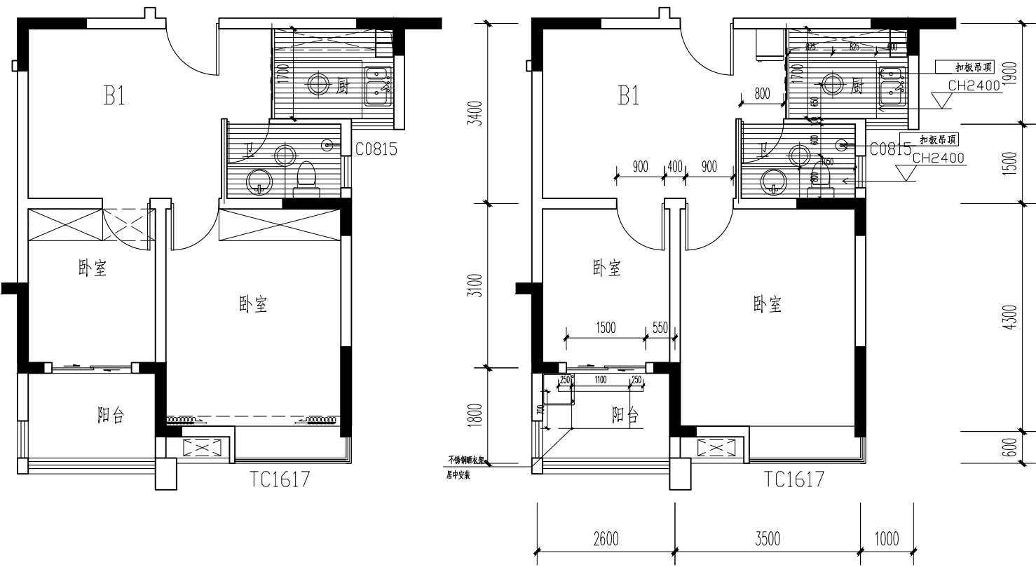
户型现状平面图 1:100
