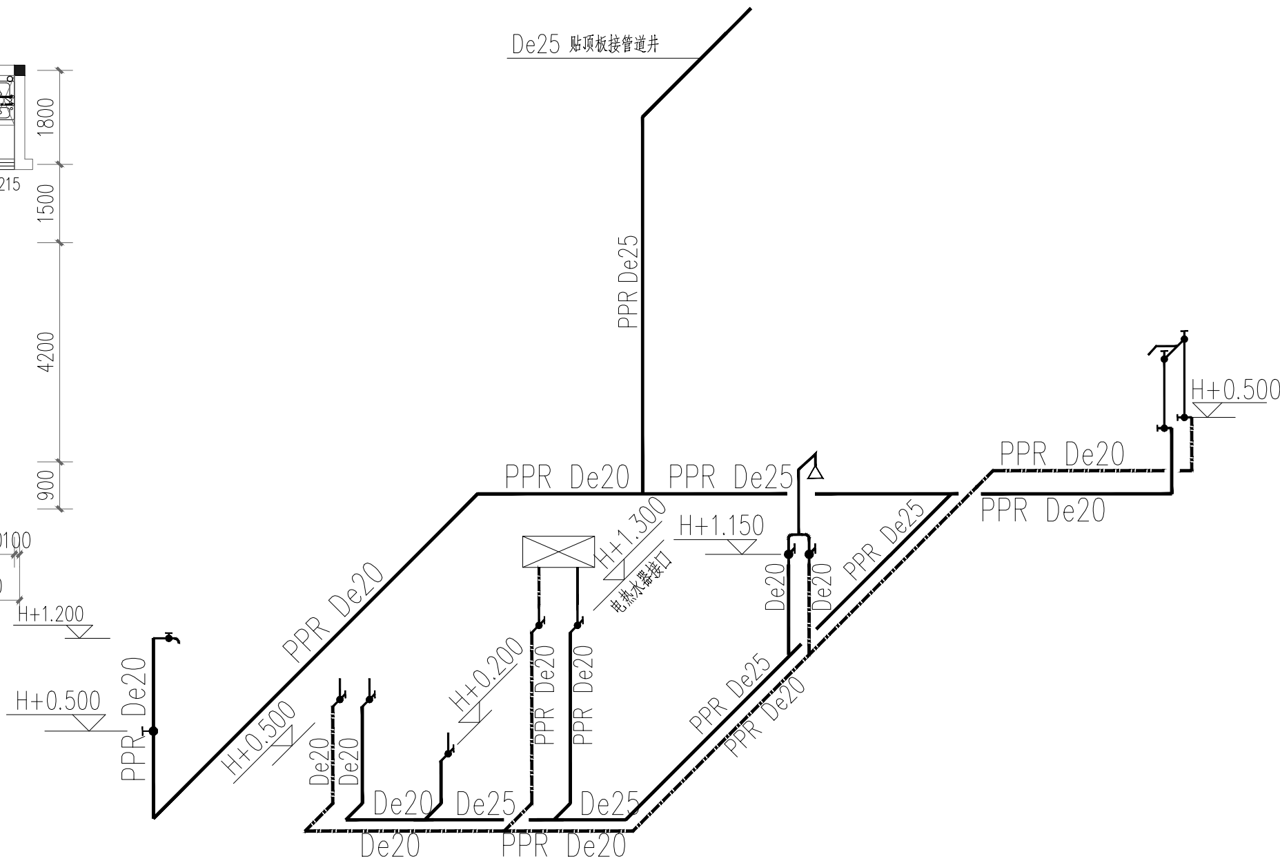
A户型厨、卫给水支管详图 1:50
