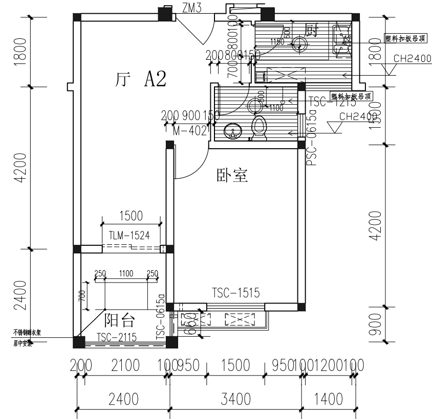
A2户型平面图 1:100
