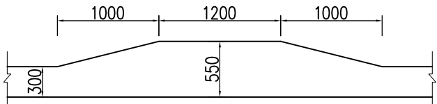
错车道设计图 1:100
