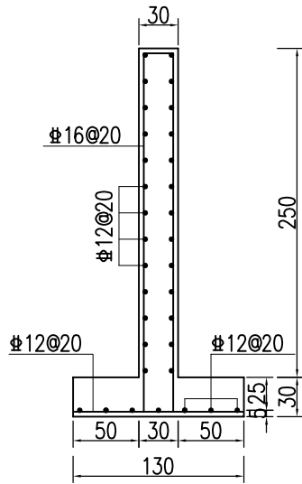
一字墙断面 1:50
