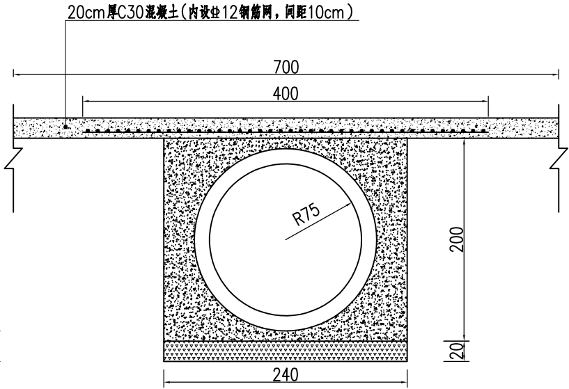
断面图 1:50 360'包封
