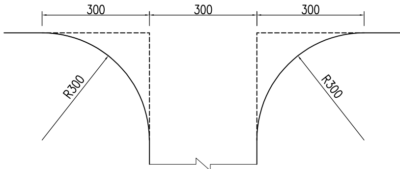
平面搭接设计图
