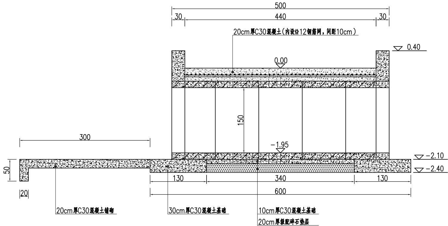
立面图 1:50
