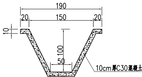
水泥渠断面设计图
