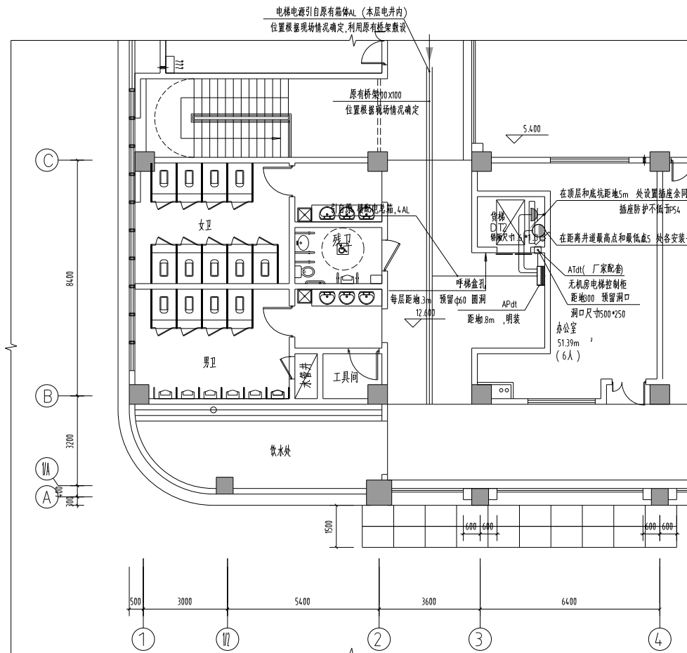
四层电梯配电平面图1:100
