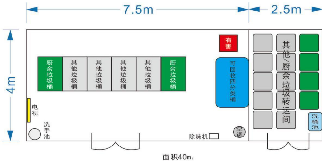
(3) 石埠湾云霞居智能垃圾分类房安装效果图（两个）
