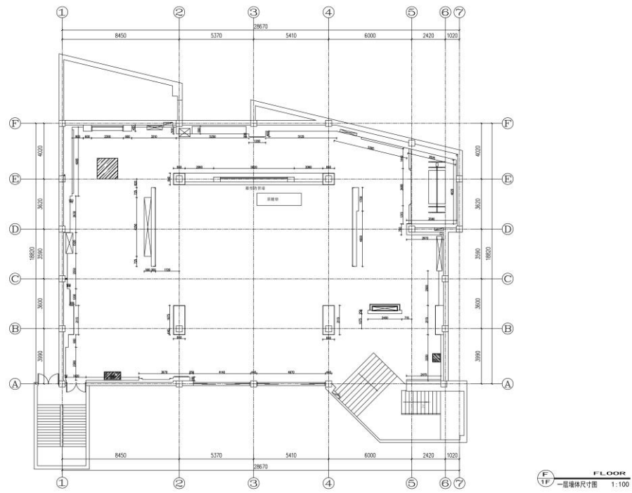
梅园新村纪念馆国共南京谈判史料陈列馆一层二层平面图
